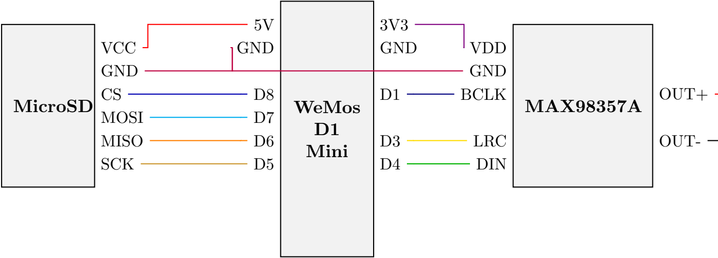
Figura 1: Esquema de interconexiones entre WeMos D1 Mini, lector MicroSD, amplificador I²S MAX98357A y altavoz.
