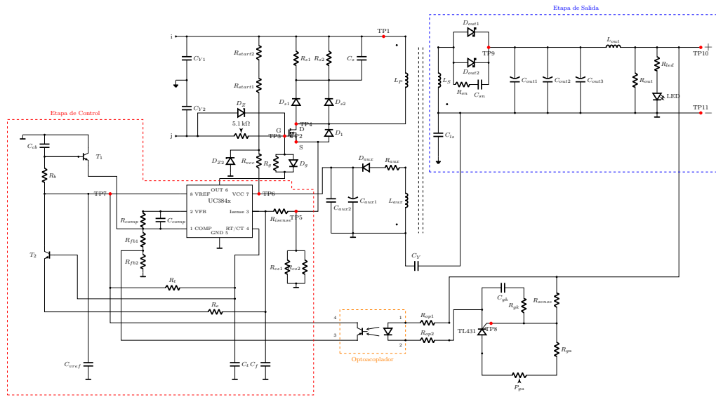
Figura 1: Esquema eléctrico básico de la etapa de conmutación (Topología Flyback).
