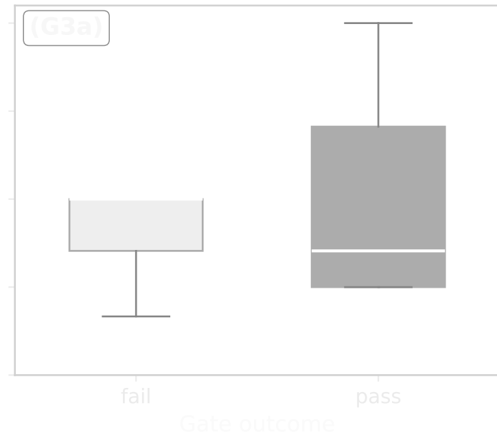
G3a (guards)
