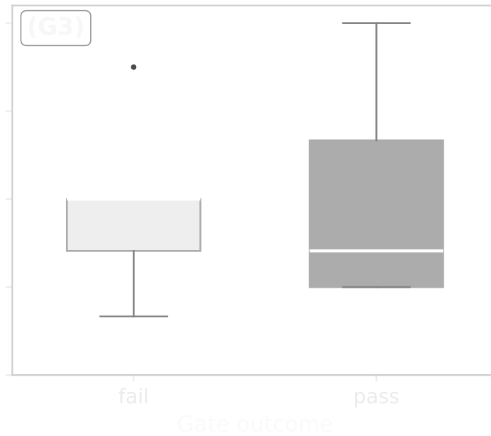
G3 (determinism)
