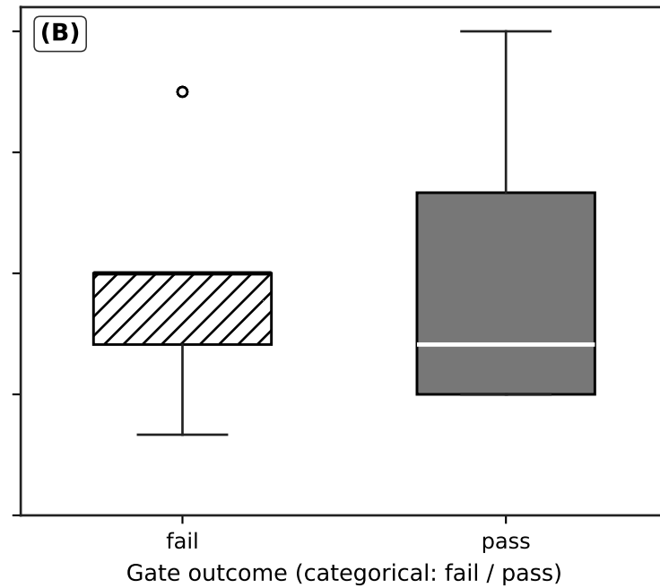
G3 (determinism)
