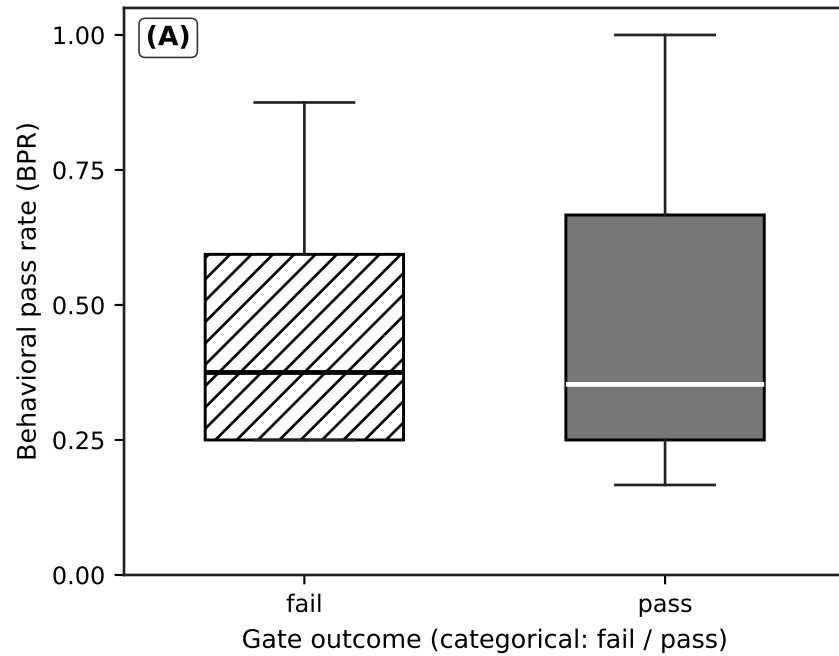
G2 (schema)
