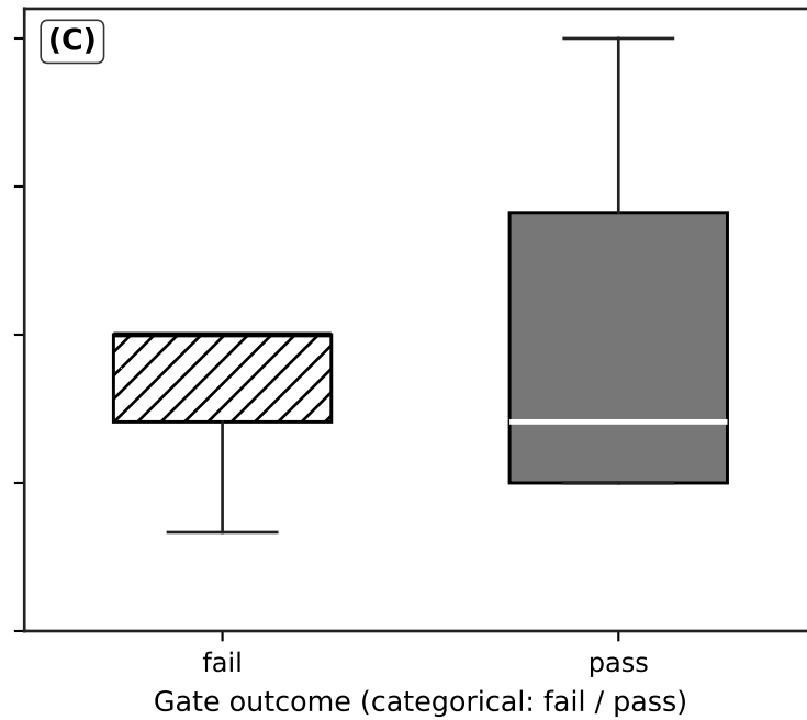
G3a (guards)
