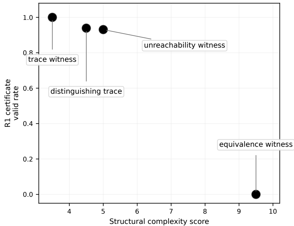
Claude Sonnet 4.5 R1
