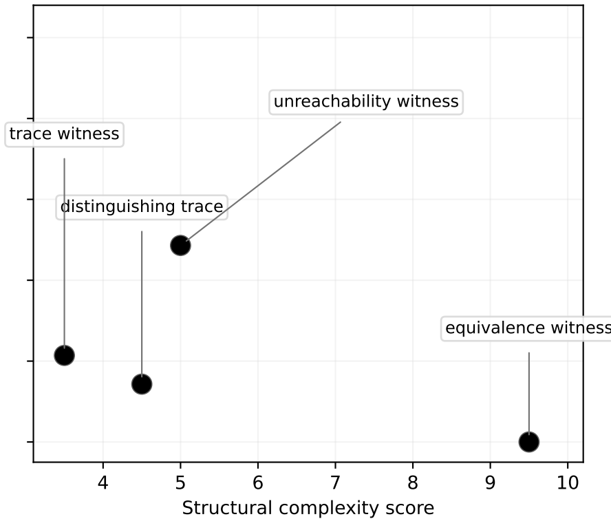
GPT-4.1 R1
