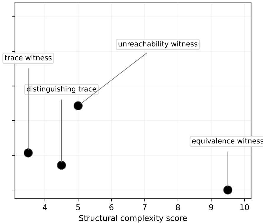
GPT-4.1 R1
