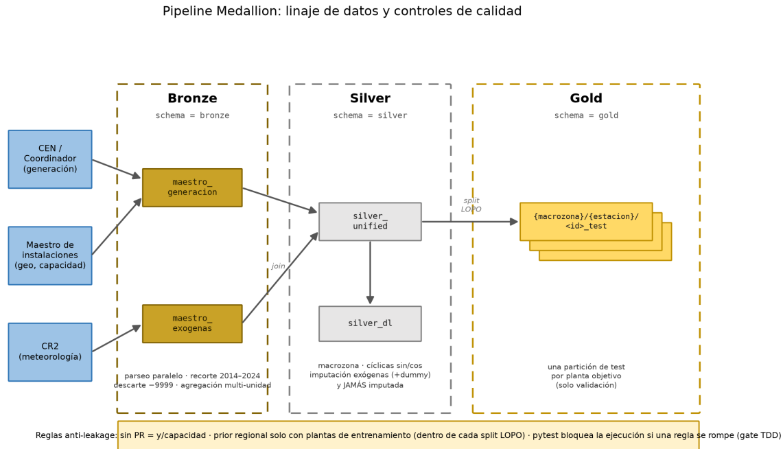
Figura 4.6: Algoritmia del proceso de preparación de datos y control de calidad.
