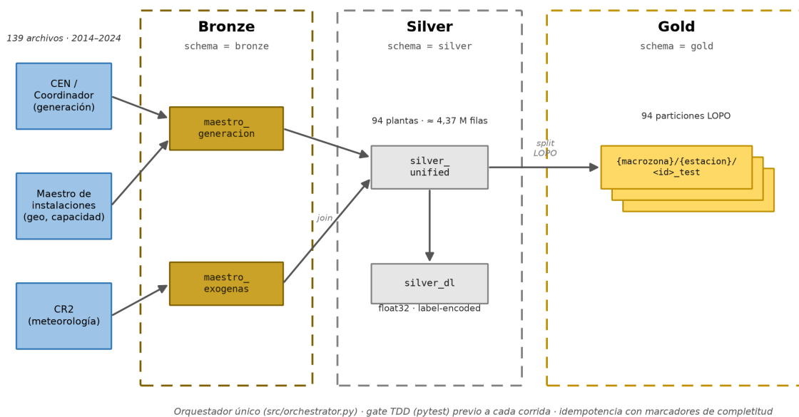
Figura 5.10: Flujo de datos implementado: Landing → Bronze → Silver → Gold, con los volúmenes reales tras la depuración.
