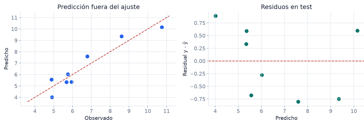
Figura 4: En una partición fija de ocho subzonas, el modelo supera la regla de referencia; las predicciones y los residuales muestran dónde se concentra el error.
