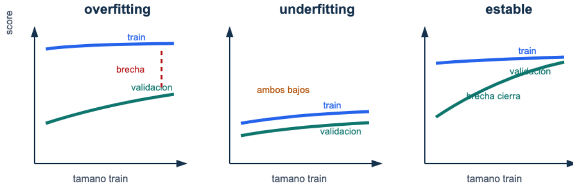
Figura 21: Curvas de aprendizaje: un caso de overfitting mantiene una brecha entre entrenamiento y validación, un caso de underfitting mantiene ambos desempeños bajos, y un caso estable cierra la brecha con más datos.
