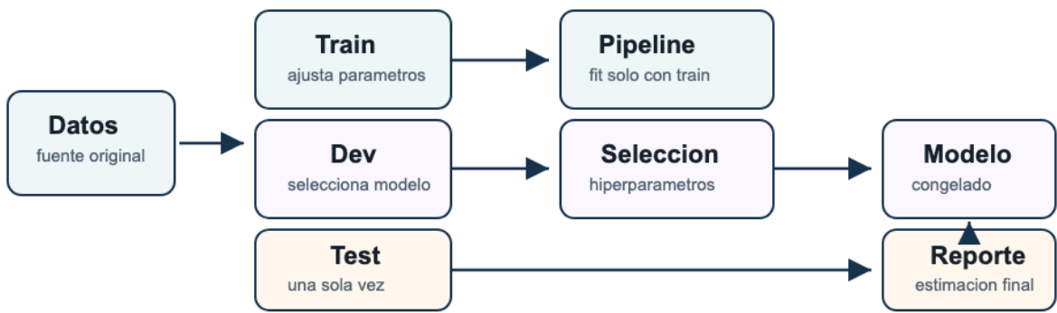
Figura 2: Flujo de validación: los datos se separan en train, dev y test; train ajusta parámetros, dev selecciona el modelo y test se usa una sola vez para reporte final.
