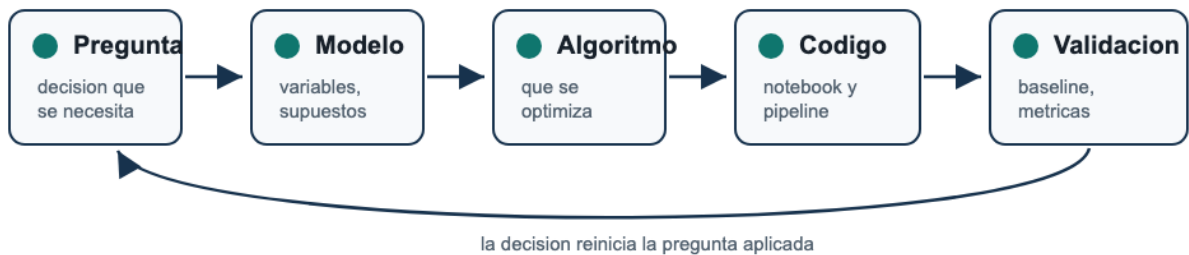
Figura 46: Ciclo de modelación aplicada del curso: pregunta aplicada, modelo matemático, algoritmo, código, validación y retorno a la pregunta.
