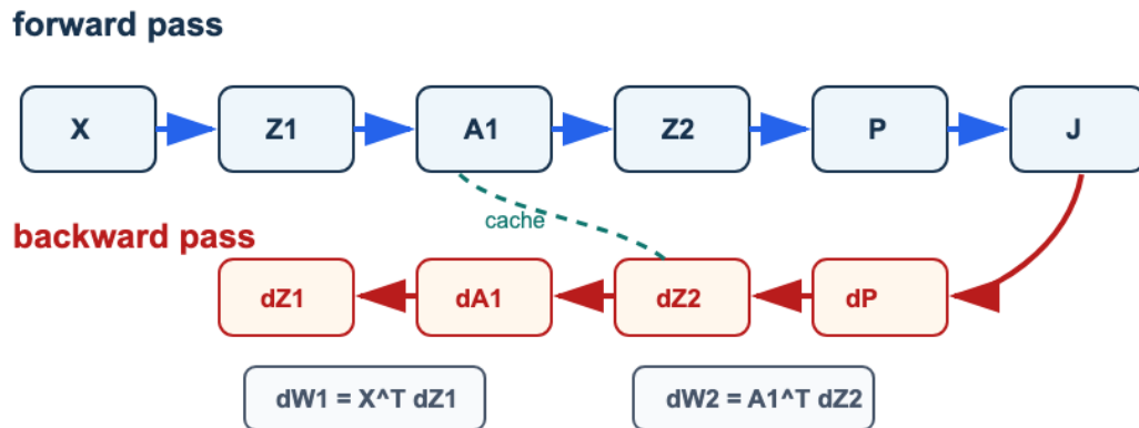
Figura 8: Backpropagation como grafo: el forward calcula X, Z1, A1, Z2, P y J; el backward propaga dJ hacia dZ2, dW2, dA1, dZ1 y dW1 usando la cache.
