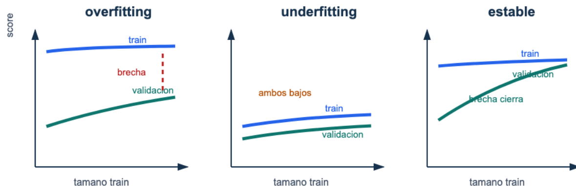
Figura 12: Curvas de aprendizaje: un caso de overfitting mantiene una brecha entre entrenamiento y validación, un caso de underfitting mantiene ambos desempeños bajos, y un caso estable cierra la brecha con más datos.
