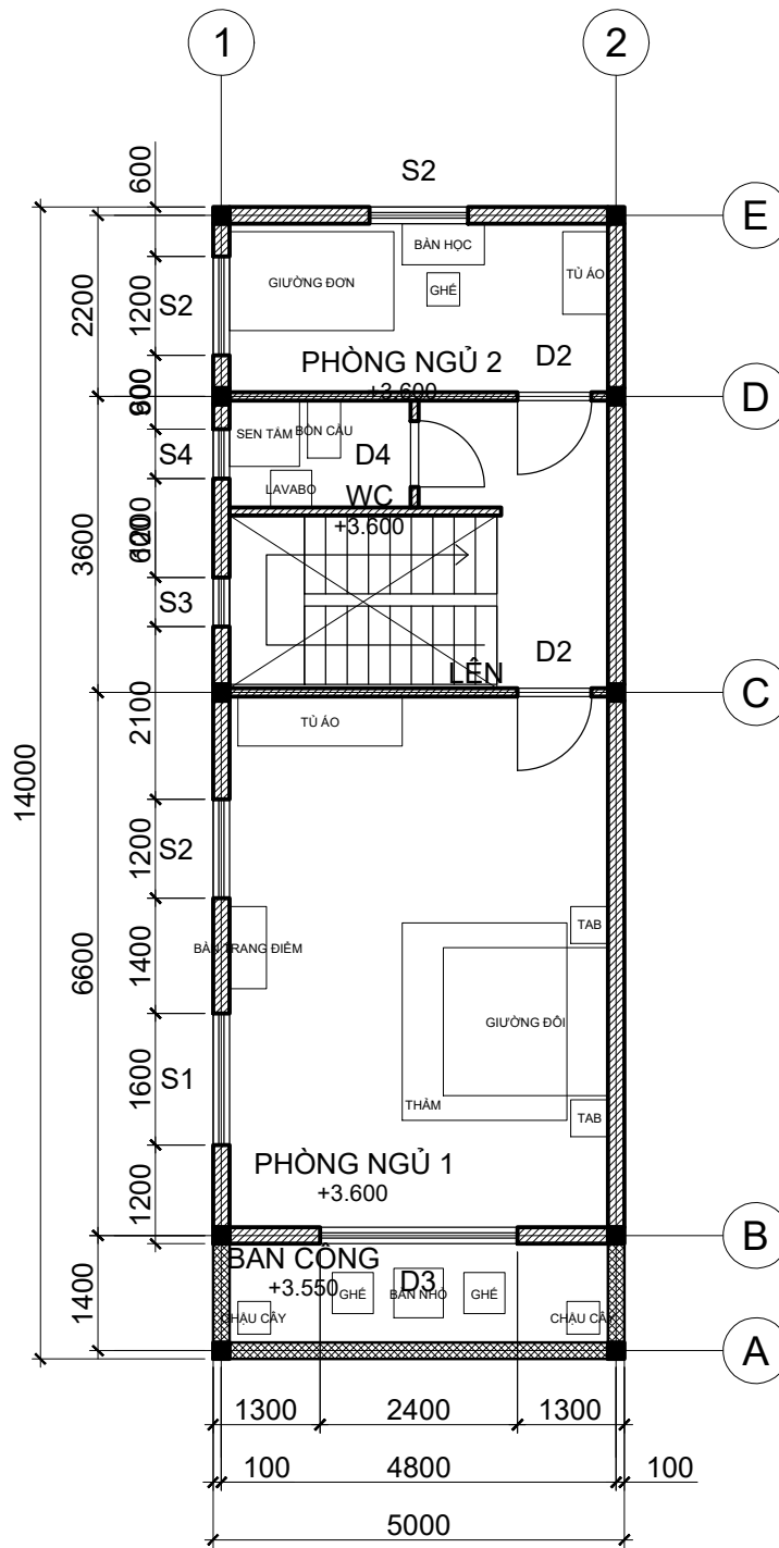
MẶT BẰNG TẦNG 2 TỶ LỆ 1/100
