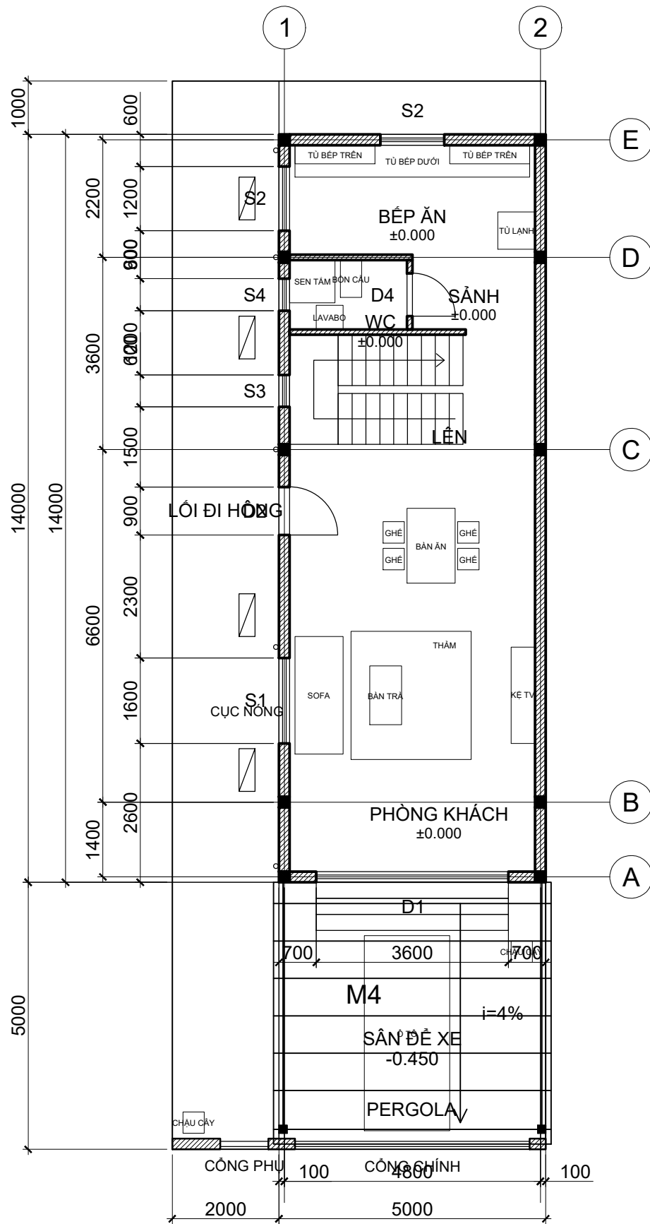
MẶT BẰNG TẦNG 1 VÀ SÂN TỶ LỆ 1/100
