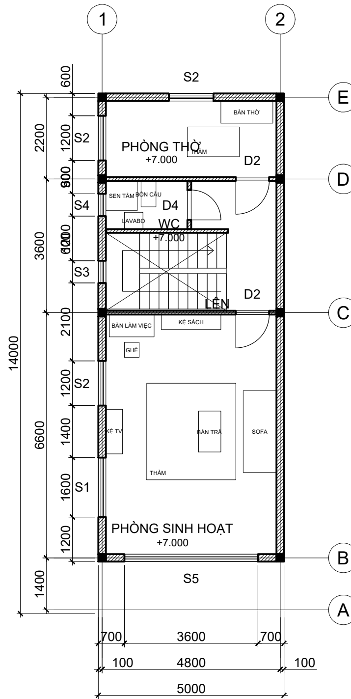
MẶT BẰNG TẦNG 3 TỶ LỆ 1/100
