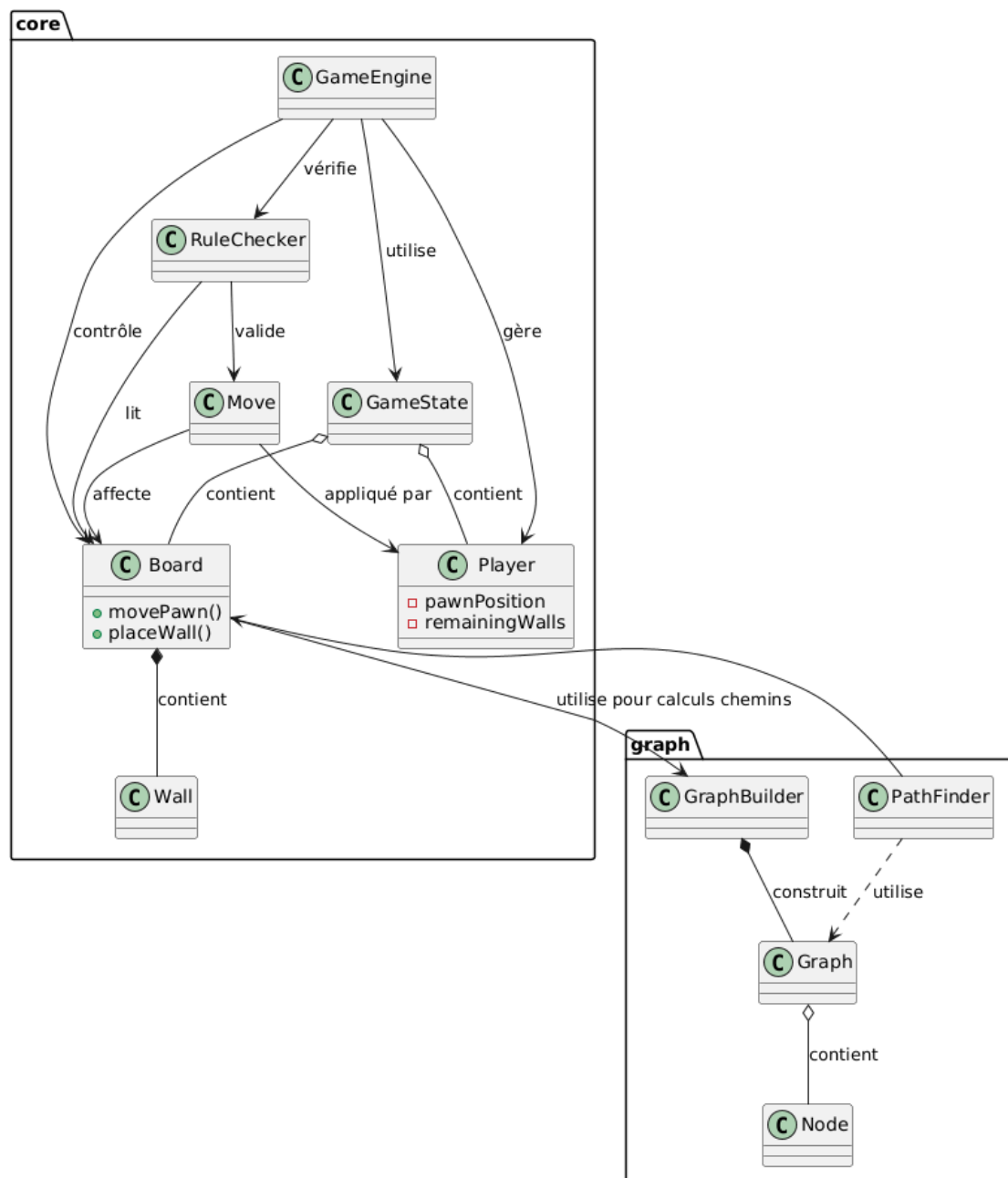
FIGURE 6 – Schéma d'UML core + graph en détaillé
