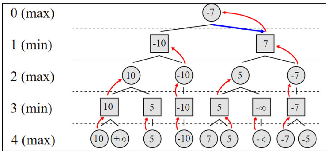
FIGURE 3 – Exemple de MiniMax
