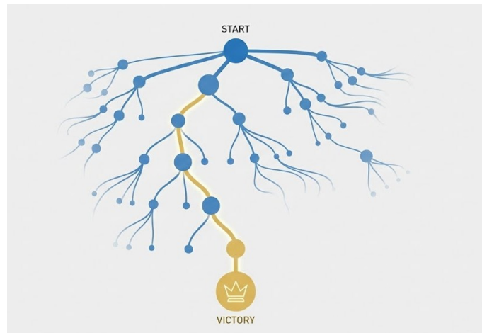
FIGURE 4 – MCTS Représentation
