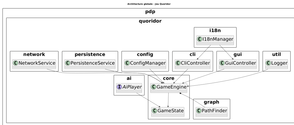
FIGURE 5 – Schéma global de l'architecture
