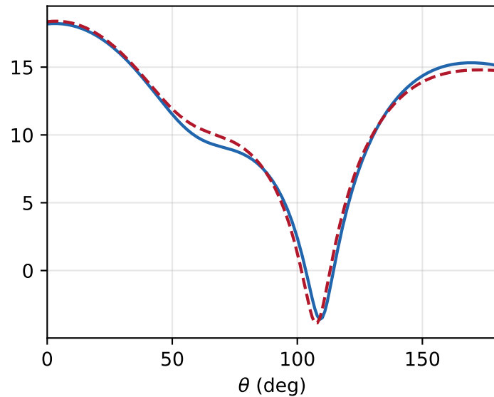
Fichera corner
