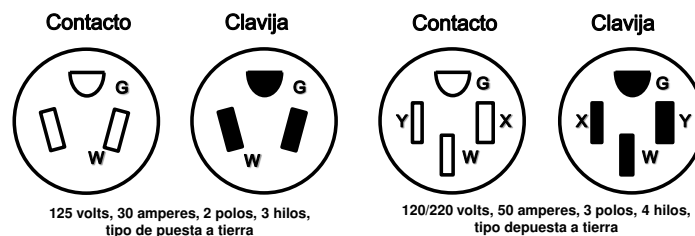
Figura 552-44(c)(1).- Configuraciones para contactos y clavijas del tipo con puesta a tierra.
