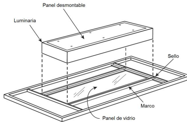
Figura 516-6(c)(a).- Ejemplo de una luminaria montada fuera del área de pulverización, mantenida y reparada desde fuera del área de pulverización.
