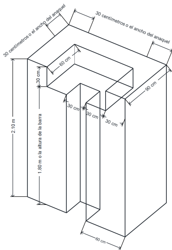
Figura 410-2.- Espacio de almacenamiento del clóset.
