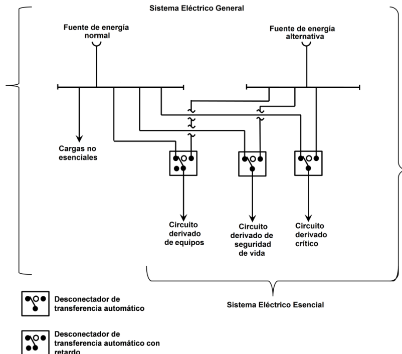
Figura 517-30 (a).- Requisito mínimo de tres desconectores de transferencia para hospitales y establecimientos para la atención médica de pacientes ambulatorios, con una demanda máxima superior a 150 kVA de la carga conectada a los tres circuitos derivados.
