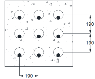
Detalle 4 675 x 675 milímetros Banco de ductos eléctricos Nueve ductos eléctricos
