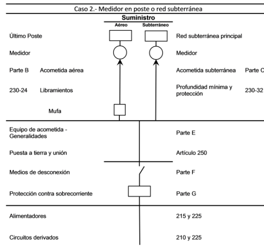
Figura 230-1.- Acometidas
