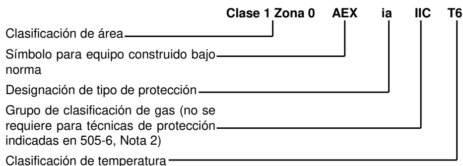
NOTA Figura 505-9(c)(2).- Marcado del equipo de zona.
