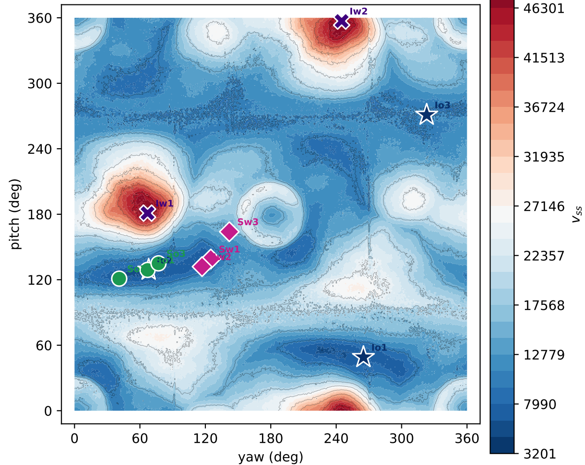
Bunny 69k: TOMO_CPU v_{ss} landscape
