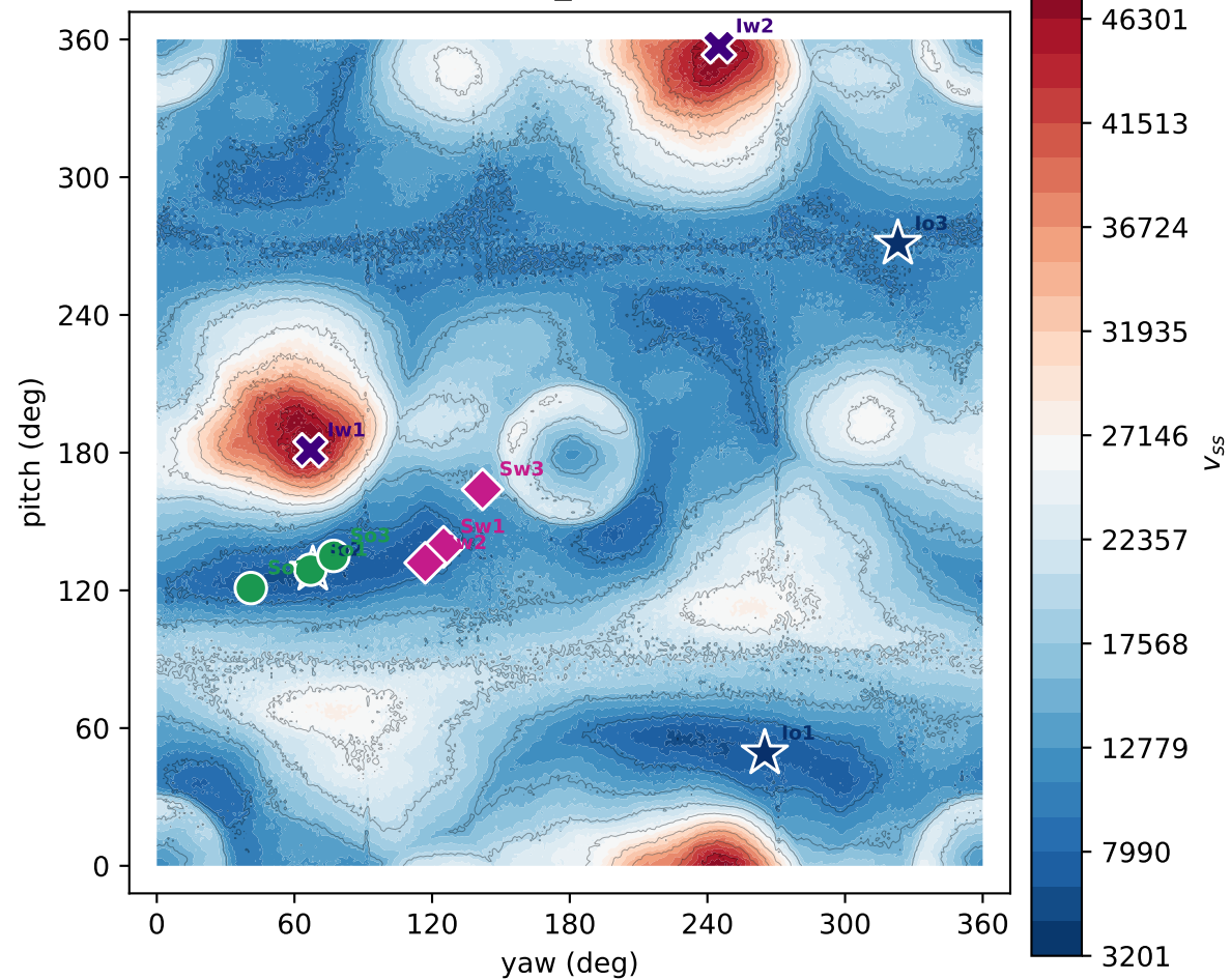
Bunny 69k: TOMO_INT3 v_{ss} landscape
