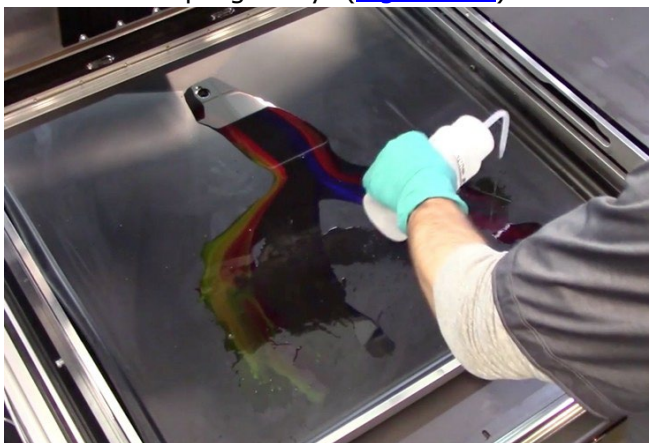
Figure 4-4 Pour Maintenance Fluid
