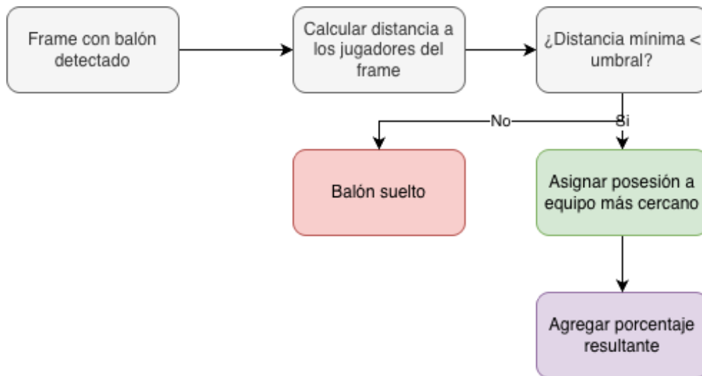
Figura 5.13: Diseño de la estimación de posesión.
