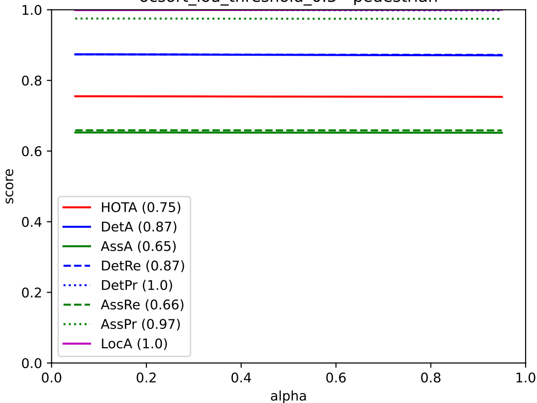
ocsort_iou_threshold_0.3 - pedestrian
