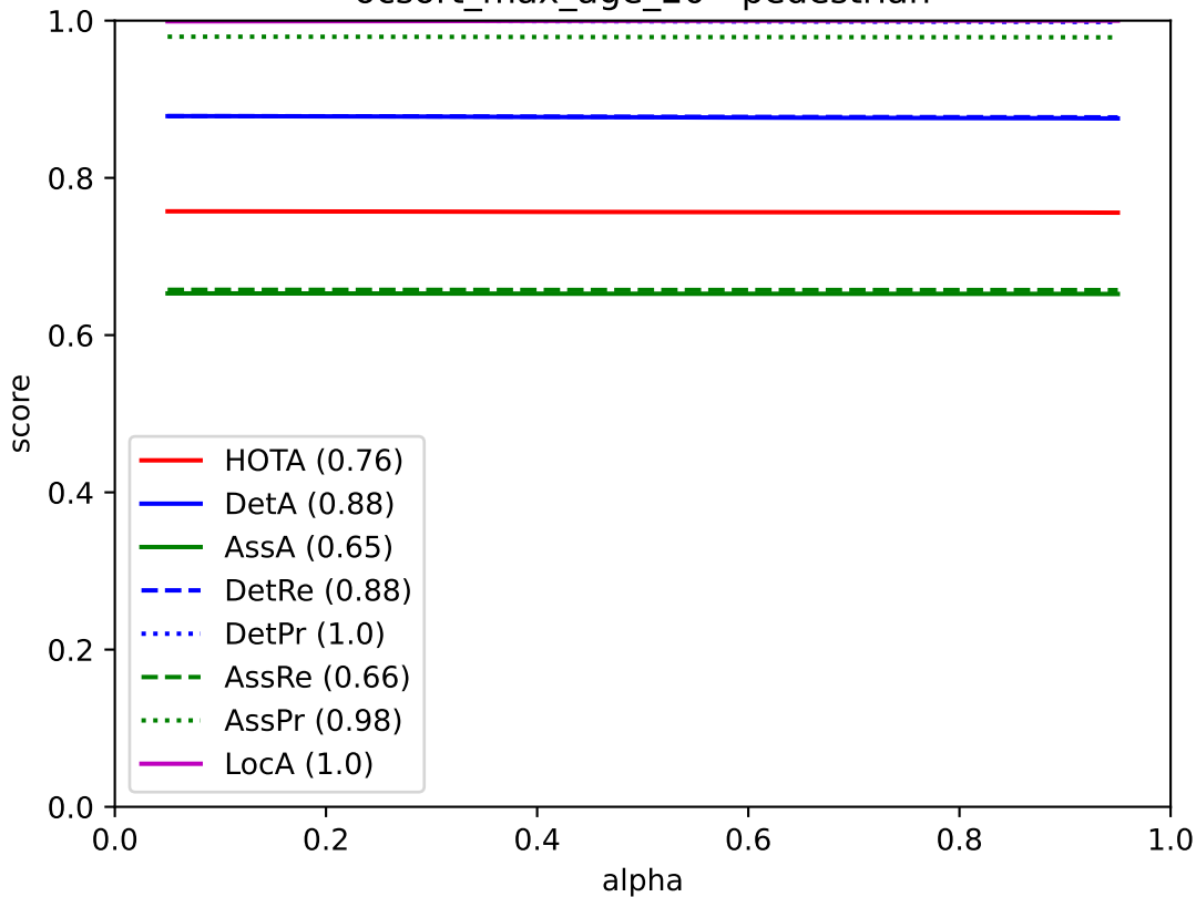
ocsort_max_age_20 - pedestrian
