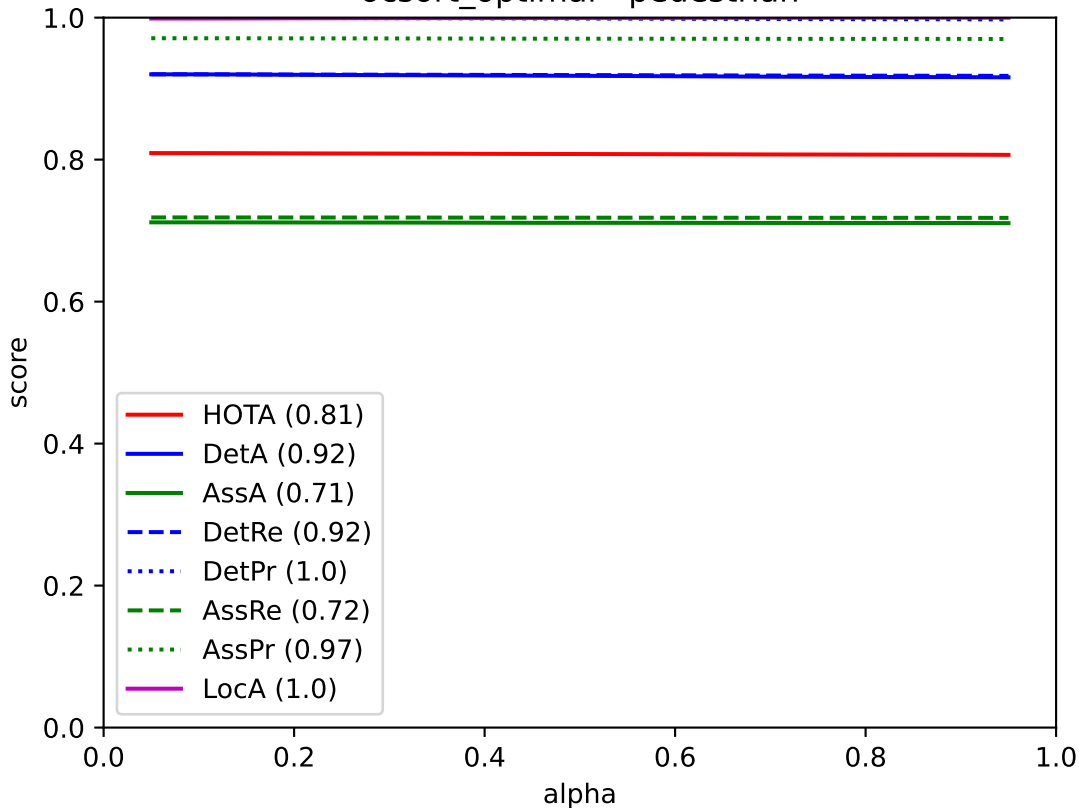
ocsort_optimal - pedestrian
