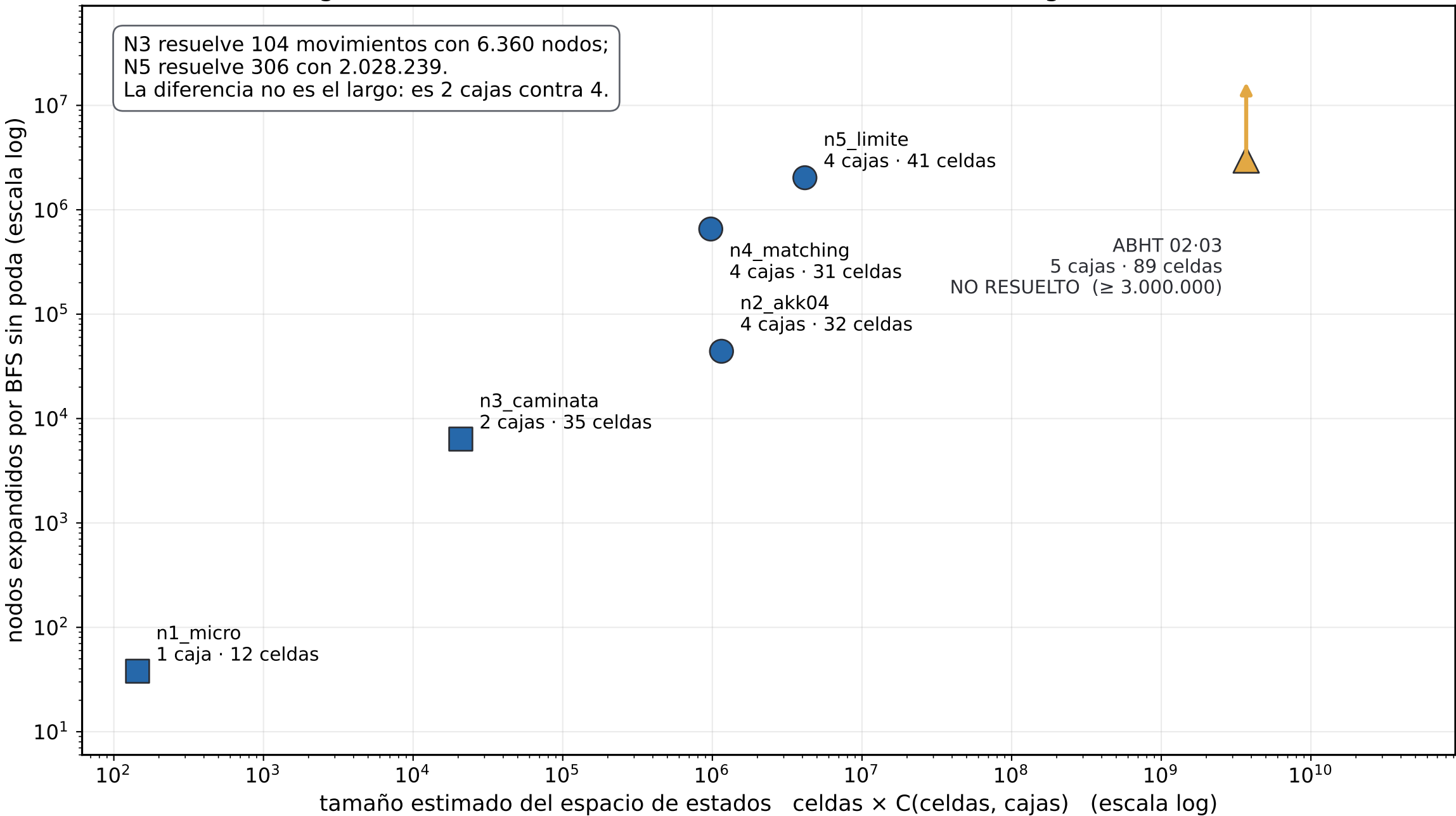
Figura 4 — El muro: el límite es combinatorio, no de largo de solución
