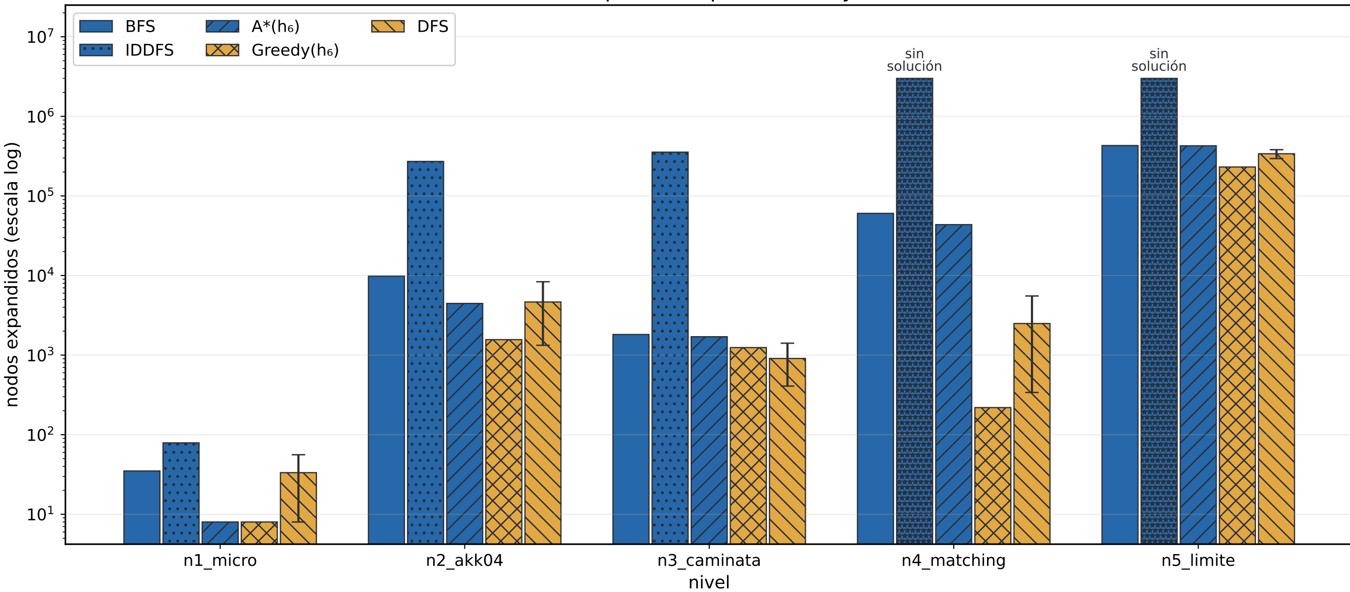
Nodos expandidos por método y nivel
