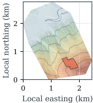
Voellmy real terrain \mu = 0.2, \xi = 2000 \text{ m s}^{-2}
