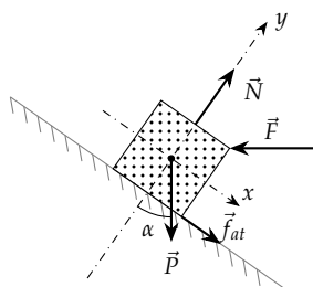
Figura 7.16: Referencial para a determinação da força normal.
