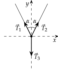
Figura 6.54: Diagrama de forças para o nó.
