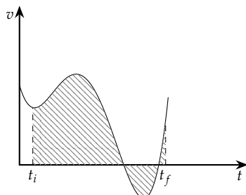
Figura 3.28: Podemos utilizar a área para determinar o deslocamento em um caso mais complexo, onde a velocidade varia arbitrariamente.
