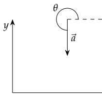
Figura 5.13: Decomposição do vetor aceleração.
