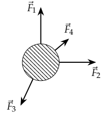
Figura 6.13: Corpo sujeito a um conjunto de forças que não se encontram em equilíbrio.
