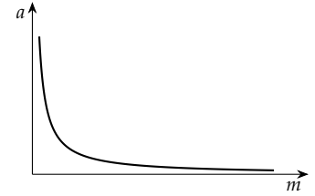
Figura 6.6: A relação entre a e m é a de que a primeira é proporcional ao inverso da segunda.
