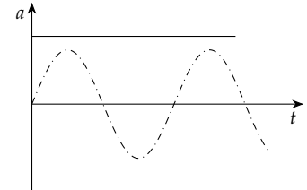
Figura 3.24: Em um gráfico a \times t , um movimento com aceleração constante corresponde a uma linha horizontal, como a linha cheia no gráfico acima. Já no caso de um sistema massa-mola, um corpo oscila devido à força exercida pela mola e devido à sua própria inércia, o que implica em uma aceleração dada por a(t) = A\omega^2 \sin(\omega t) — onde A representa a amplitude de oscilação e \omega a frequência angular, que está relacionada à frequência de oscilação —.
