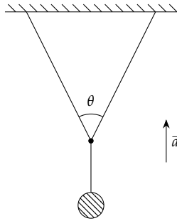
Figura 6.56: Corpo em repouso suspenso por cordas, submetido a uma aceleração vertical para cima.
