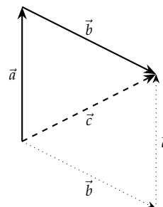
Figura 4.5: Soma de dois vetores através da “regra do paralelogramo”.
