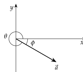
Figura 4.35: Vetor \vec{a} em relação aos eixos do sistema de referência, mostrando também o ângulo \theta entre o vetor e o eixo x , medido no sentido anti-horário.
