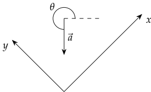
Figura 5.14: Uma escolha ruim do sistema de referência fará com que ambas as componentes do vetor aceleração sejam não nulas, o que implica em tratar ambos os eixos como movimentos acelerados.
