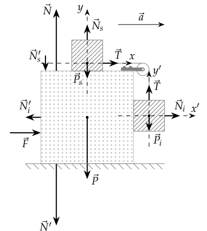
Figura 6.60: Conjunto de blocos que sofre uma aceleração para a direita: a aceleração do sistema é tal que o bloco suspenso se mantém equilibrado no eixo y' . Não há atrito entre os blocos, ou entre o bloco maior e o piso.
