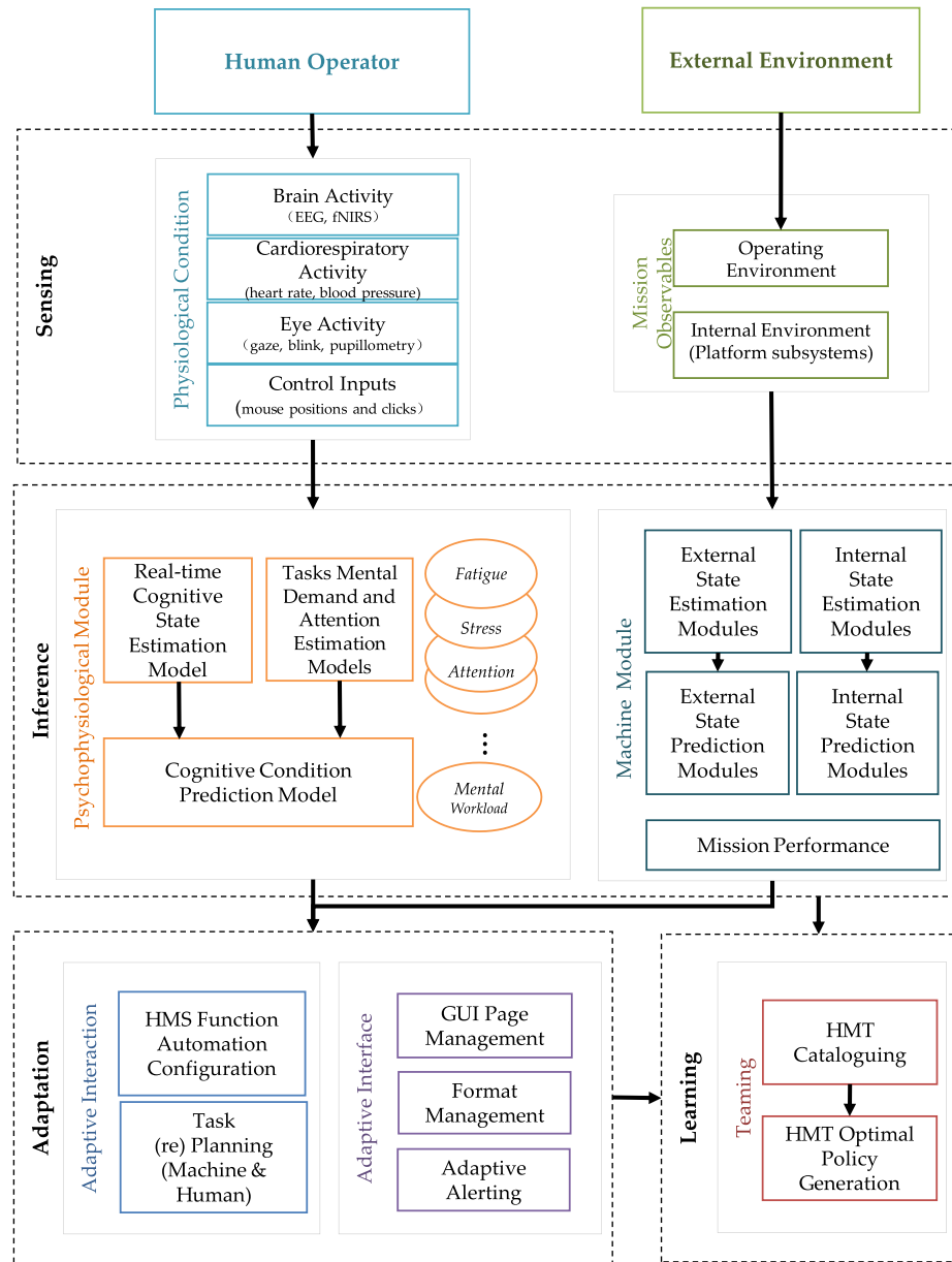
Fig. 17. CHMI 2 framework [85].
