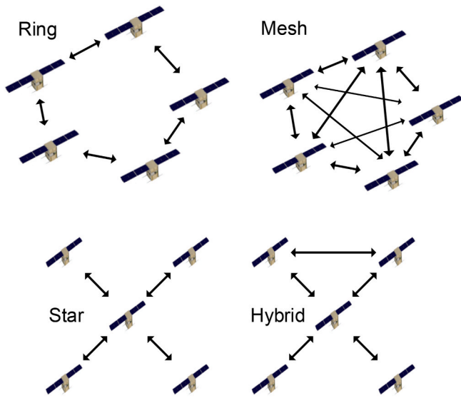
Fig. 25. Different ISL topologies [280].
