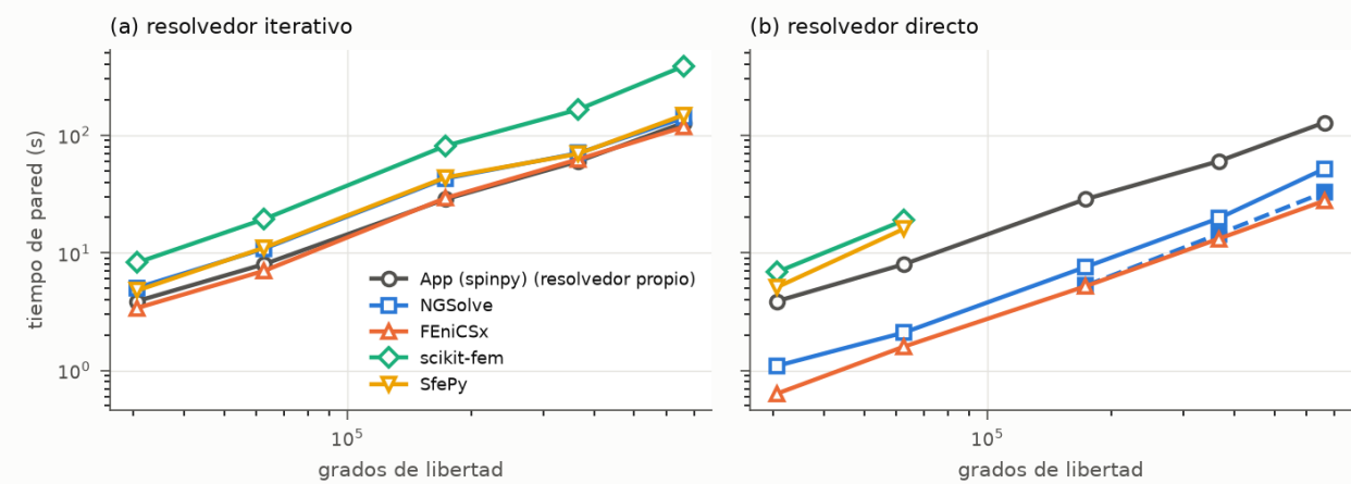
Figura 1. Tiempo de montaje y resolución del espinodoide con hexaedros frente a los grados de libertad, por motor. (a) Resolvedores iterativos; (b) directos. La app aparece en los dos paneles con su resolutor propio (LU por debajo de 6 000 GDL, CG + AMG por encima). Línea discontinua: NGSolve con su Cholesky propio.
