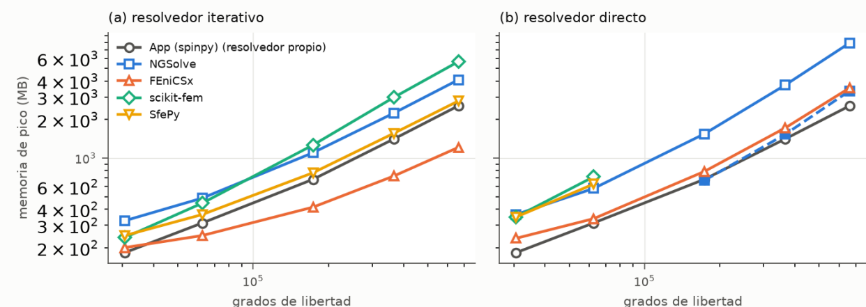
Figura 2. Memoria de pico del proceso de cálculo en los mismos casos.
