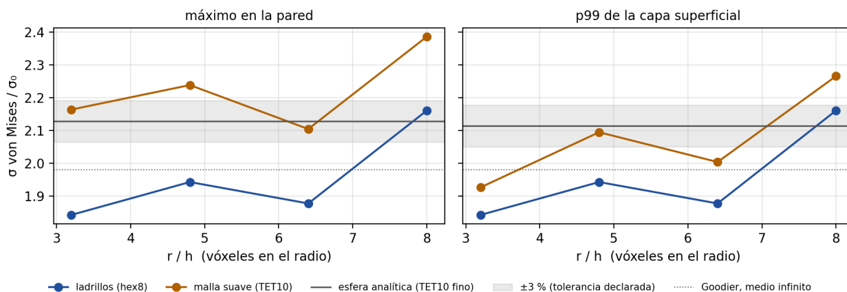
Figura 1. Pico (izquierda) y p99 de la capa superficial (derecha) de von Mises en la pared de la cavidad, normalizados por la tensión aplicada, frente a los vóxeles en el radio. La banda gris es \pm 3 % alrededor de la referencia analítica (tolerancia declarada antes de medir); la línea de puntos, Goodier en medio infinito.
