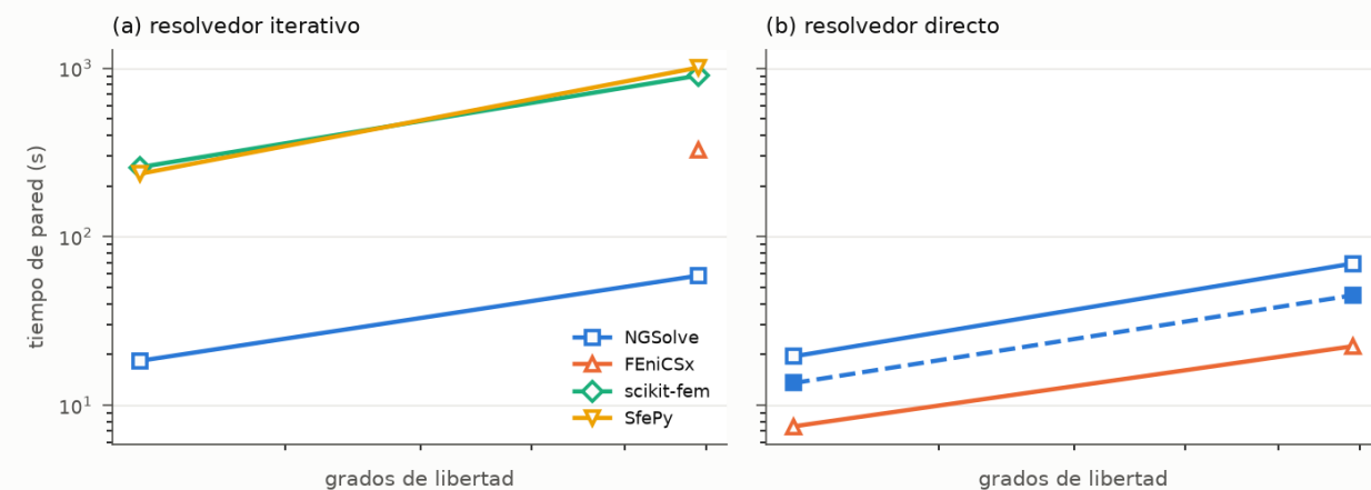
Figura 3. Figura 3. Tiempo del espinodoide con TET10. (a) Iterativos; (b) directos (línea discontinua: NGSolve con su Cholesky propio).
