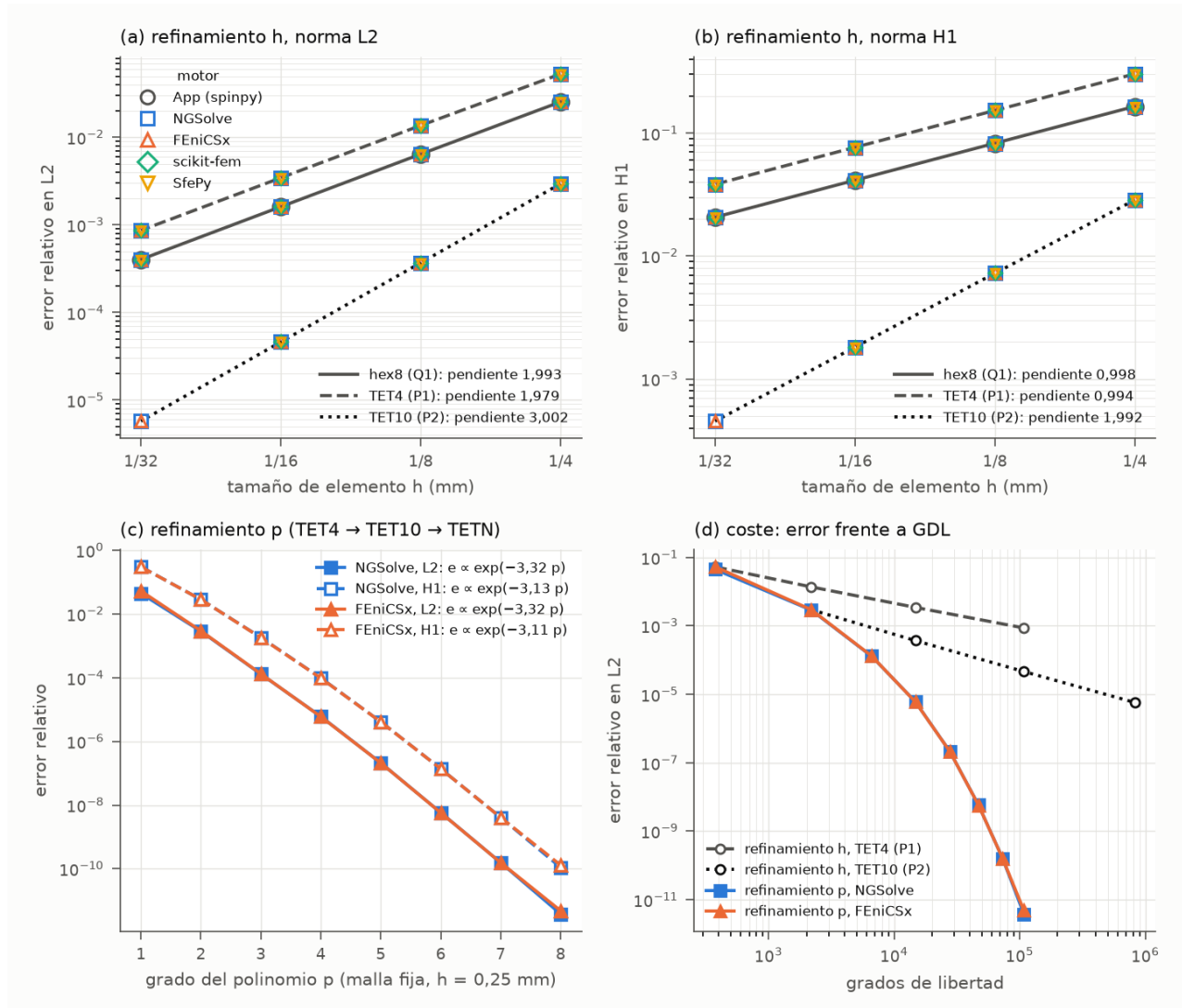
Figura 5. Figura 5. Convergencia de los motores hacia la solución exacta del cubo. (a, b) Error relativo en L2 y en la seminorma H1 frente al tamaño de elemento h (refinamiento h ), con la pendiente de mínimos cuadrados de cada elemento; los marcadores de los cinco motores se superponen porque resuelven el mismo problema discreto. Las pendientes teóricas son k + 1 en L2 y k en H1 ( k = 1 para hex8 y TET4; k = 2 para TET10). (c) Refinamiento p con la malla fija ( h = 0,25 mm): el logaritmo del error decrece linealmente con el grado; trazo continuo, L2; discontinuo, H1. (d) Error L2 frente a los grados de libertad: el refinamiento h da rectas en log-log y el refinamiento p , una curva que se inclina cada vez más (convergencia exponencial).
