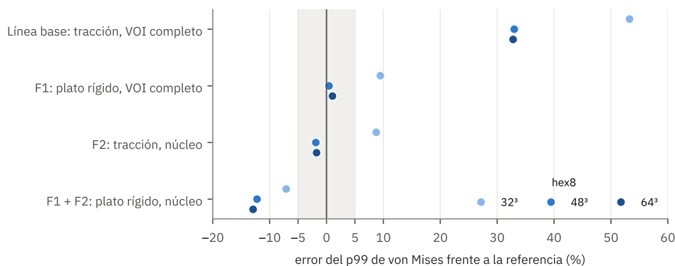
Figura 4. Error del p99 de von Mises frente a la referencia. El plato rígido sobre el VOI completo y el núcleo con tracción quedan cerca de cero a 48 3 y 64 3 ; el núcleo con plato lo subestima entre un 7 y un 13 %.
