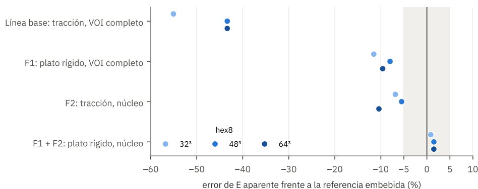
Figura 3. Error del E aparente frente a la referencia embebida, por método y resolución. Banda gris: \pm 5\% . Solo la combinación de plato y núcleo cae dentro de la banda en las tres resoluciones.
