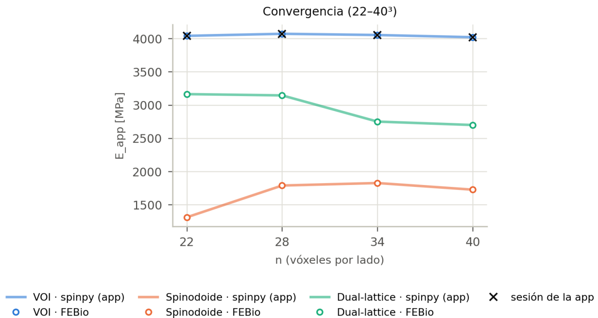
Figura 8. E_{app} frente a la resolución. Líneas: spinpy; círculos: FEBio; cruces: la serie que guardó la sesión (solo el VOI).
