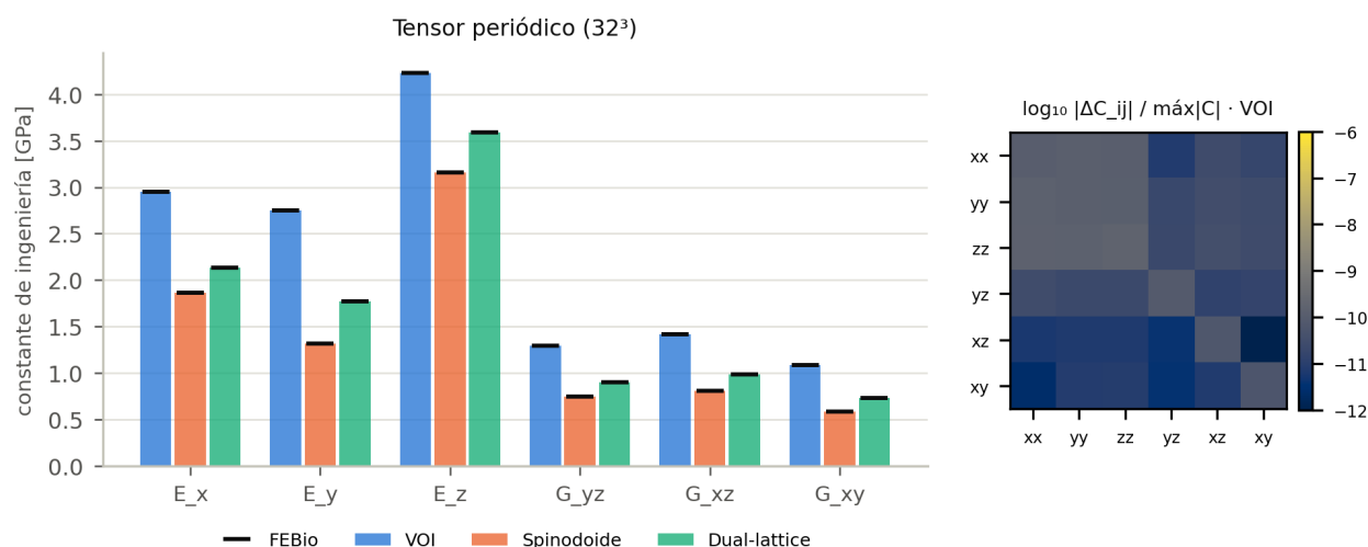
Figura 7. Constantes de ingeniería del tensor periódico: barras spinpy, trazos FEBio. A la derecha, \log_{10} de la diferencia entrada a entrada del tensor del VOI, relativa a su mayor entrada.
