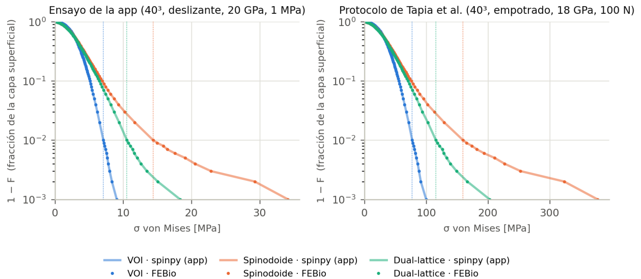
Figura 6. Distribución de von Mises en la capa superficial, de la que sale el p99 citable (líneas punteadas): excedencia 1 - F , 111 cuantiles hazen. Líneas: spinpy; puntos: FEBio. Eje cortado en p99,9.
