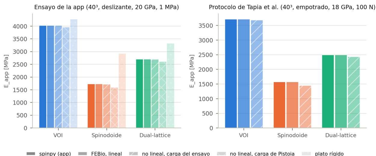
Figura 10. Módulo aparente de cada estructura: spinpy, FEBio lineal, FEBio no lineal a la carga del ensayo y a la de Pistoia, y plato rígido.
