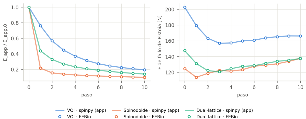
Figura 9. Fallo progresivo. Izquierda: rigidez relativa al paso 0. Derecha: carga de fallo de Pistoia de la estructura ya dañada. Líneas: spinpy; círculos: el mismo algoritmo con FEBio como solver.
