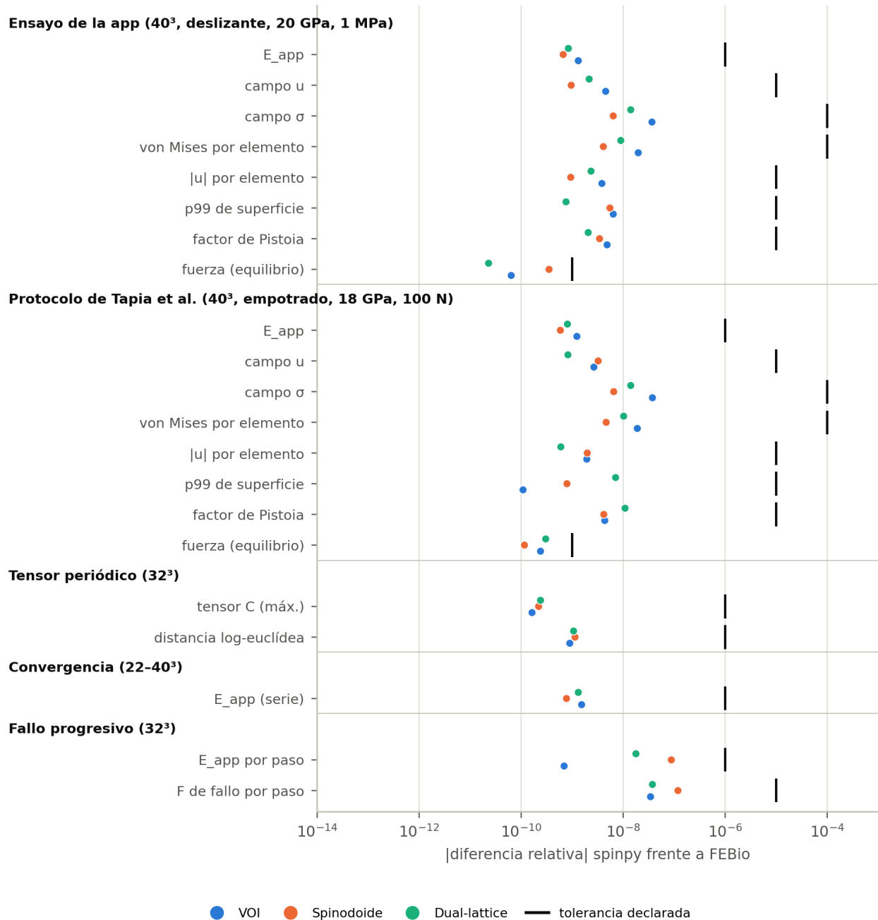
Figura 1. Diferencia relativa entre spinpy y FEBio en cada magnitud y cada análisis (puntos, uno por estructura), frente a la tolerancia declarada (trazo negro). Escala logarítmica. En el fallo progresivo y la convergencia se muestra el peor paso o la peor resolución.
