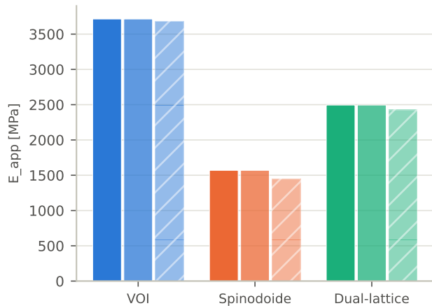
Protocolo de Tapia et al. (40 3 , empotrado, 18 GPa, 100 N)
