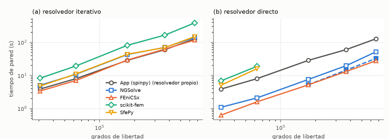
Figura 1. Tiempo de montaje y resolución del espinodoide con hexaedros frente a los grados de libertad, por motor. (a) Resolvedores iterativos; (b) directos. La app aparece en los dos paneles con su resolutor propio (LU por debajo de 6 000 GDL, CG + AMG por encima). Línea discontinua: NGSolve con su Cholesky propio.
