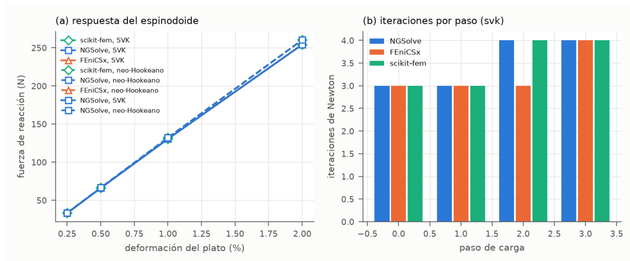
Figura 6. (a) Fuerza de reacción del espinodoide frente al acortamiento del plato, por motor y material: las curvas se superponen. (b) Iteraciones de Newton por paso con St. Venant-Kirchhoff.
