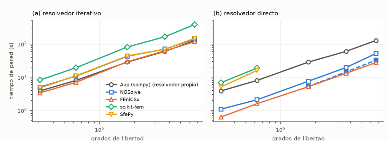
Figura 1. Tiempo de montaje y resolución del espinodoide con hexaedros frente a los grados de libertad, por motor. (a) Resolutores iterativos; (b) directos. La app aparece en los dos paneles con su resolutor propio (LU por debajo de 6 000 GDL, CG + AMG por encima). Línea discontinua: NGSolve con su Cholesky propio.
