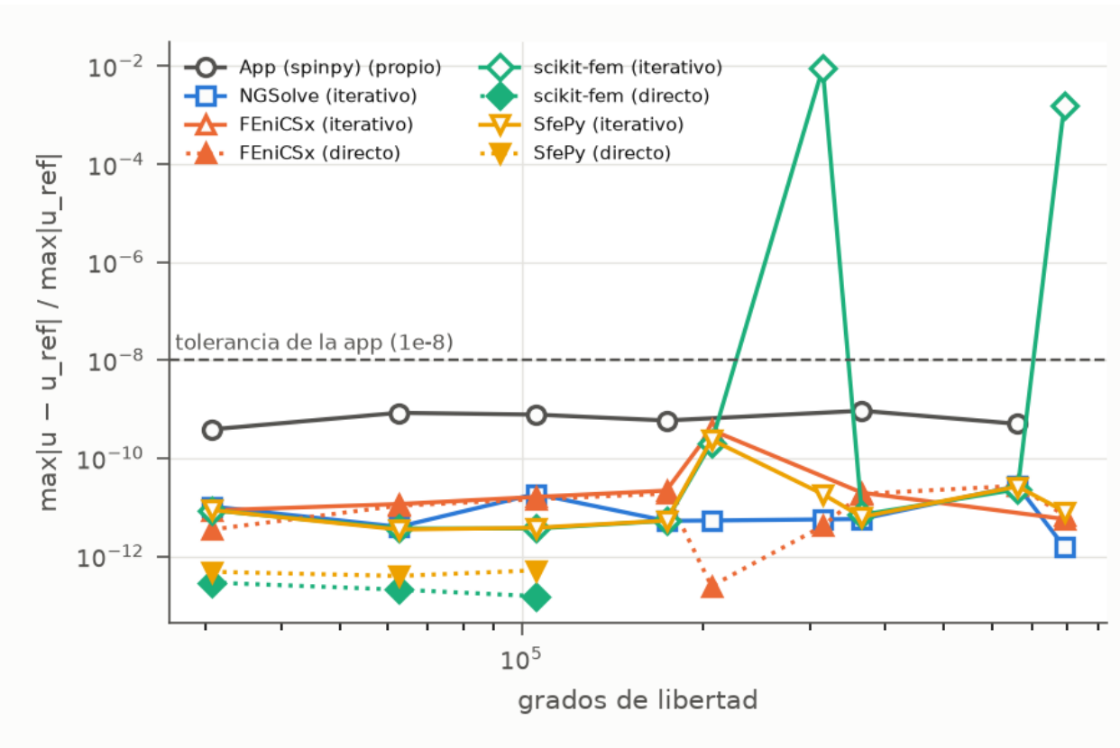
Figura 5. Diferencia máxima de desplazamientos de cada motor y resolvidor frente a la referencia directa del caso, en todos los casos lineales del espinodoide y de la cavidad. Línea discontinua: la tolerancia del resolvidor de la app. Los dos picos de scikit-fem son sus soluciones iterativas en las mallas TET10.
