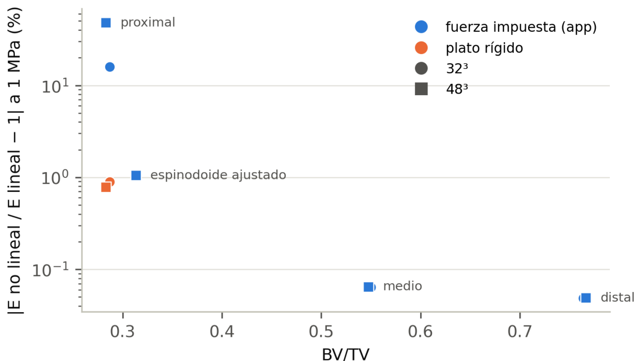
Figura 2. Pérdida no lineal de rigidez a 1 MPa frente a BV/TV. Azul: fuerza impuesta, el ensayo de la app. Naranja: plato rígido (apartado 3.3). Círculos 32^3 , cuadrados 48^3 .
