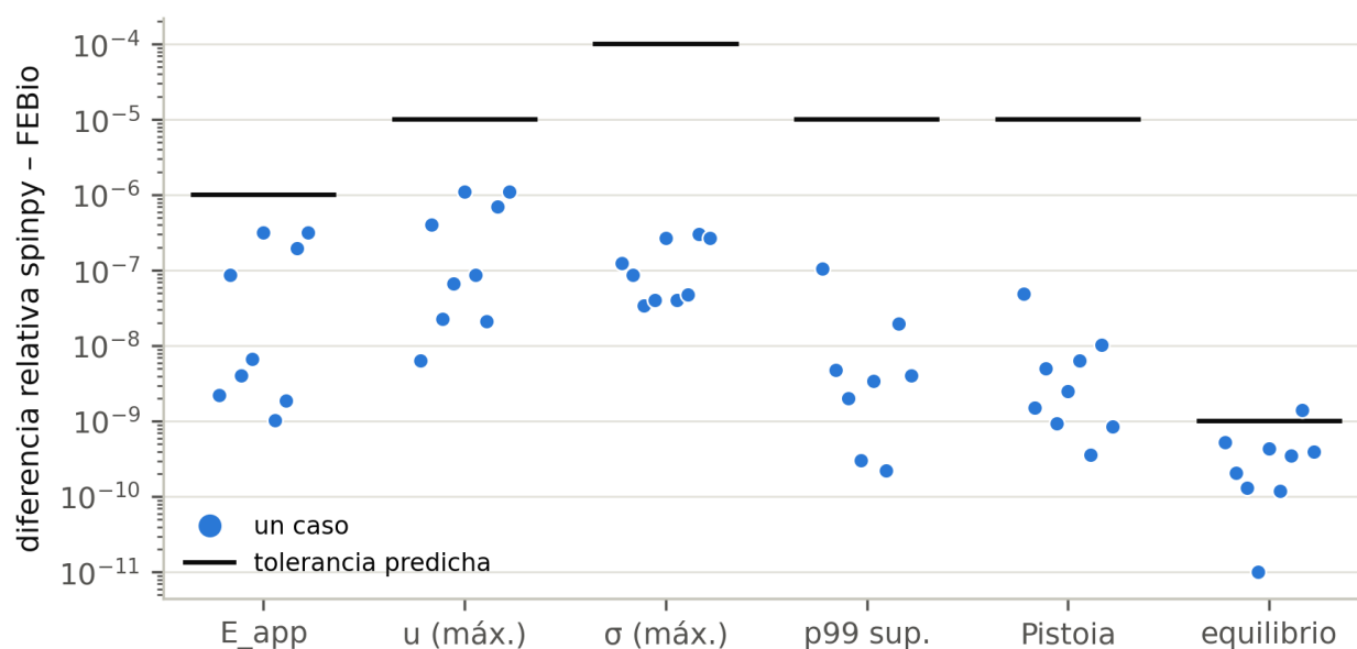
Figura 1. Diferencia relativa entre spinpy y FEBio en cada métrica y cada caso (puntos), frente a la tolerancia predicha antes de medir (trazo negro). Escala logarítmica.
