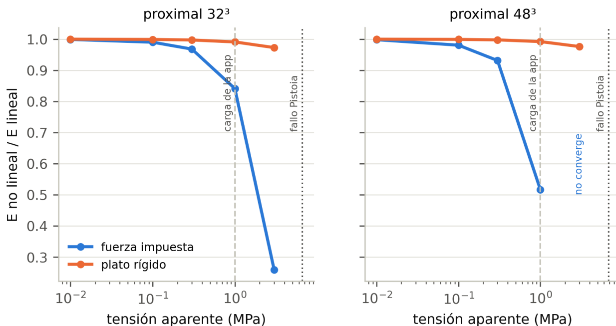
Figura 4. Rigidez no lineal / lineal frente a la tensión aparente, con fuerza impuesta (azul) y con plato rígido (naranja). Línea discontinua: carga de referencia de la app. Punteada: carga de fallo de Pistoia. Con fuerza impuesta, el proximal a 48³ no converge a 3 MPa.
