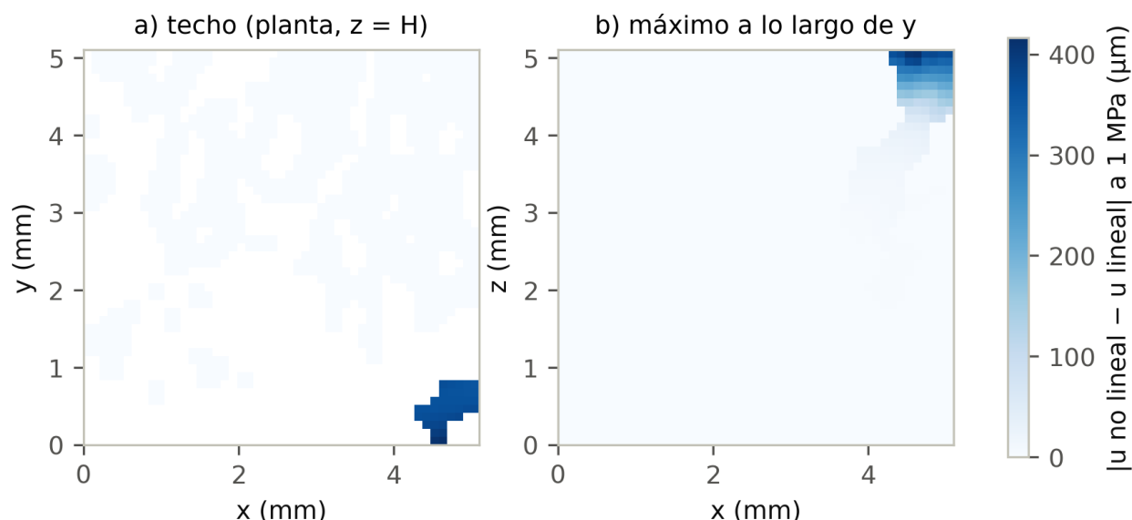
Figura 3. Desvío no lineal de cada nodo a 1 MPa en el VOI proximal a 48^3 : a) en planta, sobre la cara cargada; b) máximo a lo largo de y . Casi todo está en una esquina del techo.
