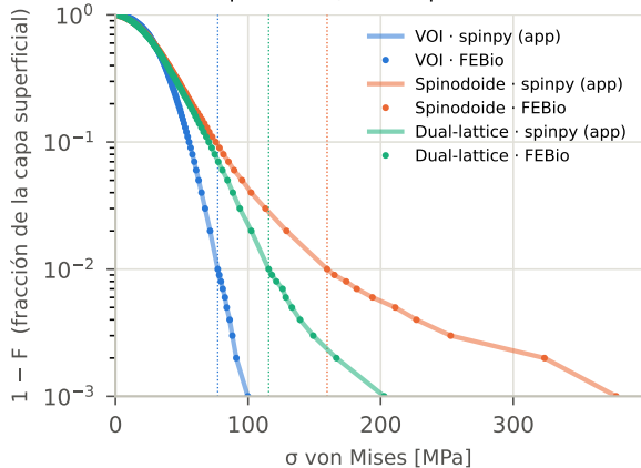
Protocolo de Tapia et al. ( 40^3 , empotrado, 18 GPa, 100 N)
