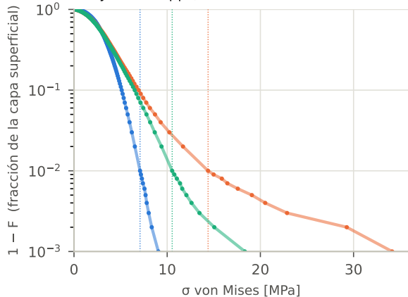
Ensayo de la app ( 40^3 , deslizante, 20 GPa, 1 MPa)
