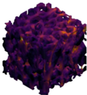
spinpy (app)
