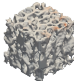
FEBio no lineal - \text{app}
