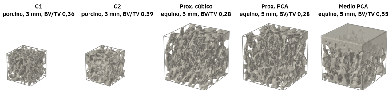
Figura 4. Los cinco VOIs, dibujados a la misma escala (superficie del hueso, remuestreada a 80^3 solo para el dibujo). Los porcinos miden 3 mm de lado y los equinos, 5 mm. La carga se aplica en el eje vertical de cada imagen.
