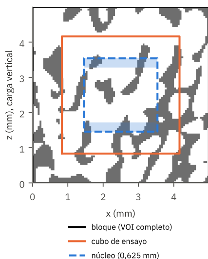
Figura 3. Corte vertical del mismo VOI, con las dimensiones reales: bloque (negro), cubo de ensayo (naranja) y núcleo a 0,625 mm de las caras (azul), con las franjas del extensómetro sombreadas. La carga es vertical.
