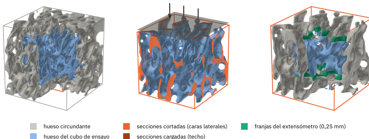
Figura 2. Los tres objetos del ensayo sobre el VOI proximal cúbico (equino), en 3D. (a) Bloque de 96^3 con un cuarto retirado para ver el cubo de ensayo (azul) dentro del hueso circundante (gris). (b) El cubo de ensayo aislado, como lo ensaya la aplicación: en naranja, las secciones de trabéculas cortadas por las caras laterales, que quedan sin apoyo; en granate, las secciones del techo, donde se aplica la carga (plato y flechas). (c) El núcleo a 0,625 mm de las caras (en azul, con un cuarto retirado) y las dos franjas del extensómetro virtual (verde) en las que se mide la deformación.
