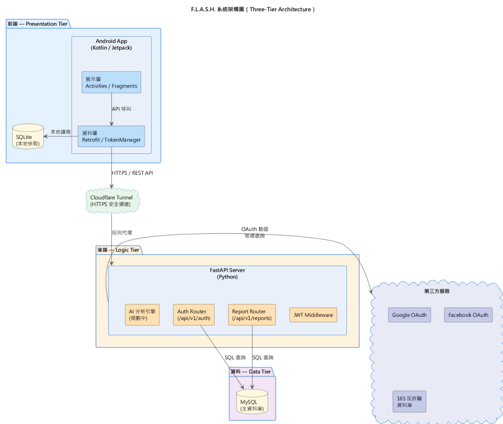
圖 2-1：閃騙俠 The F.L.A.S.H. 系統架構圖 ( Three-Tier Architecture )
