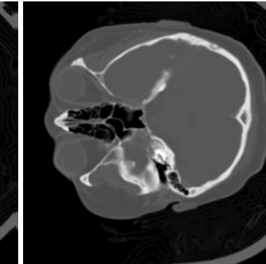
STN Affine
