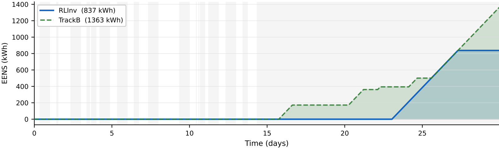
④ Cumulative Unmet Load (EENS)
