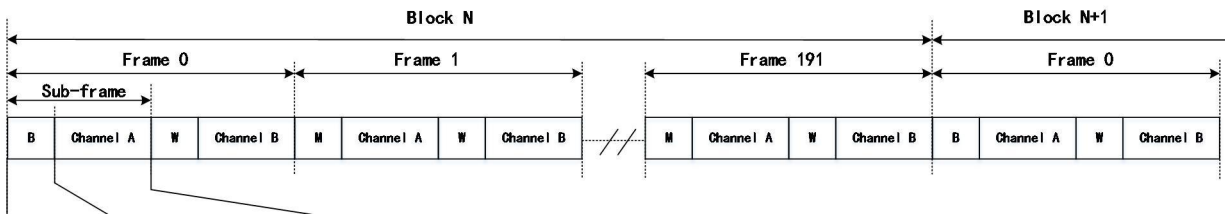
图 36-10 SPDIF 格式
