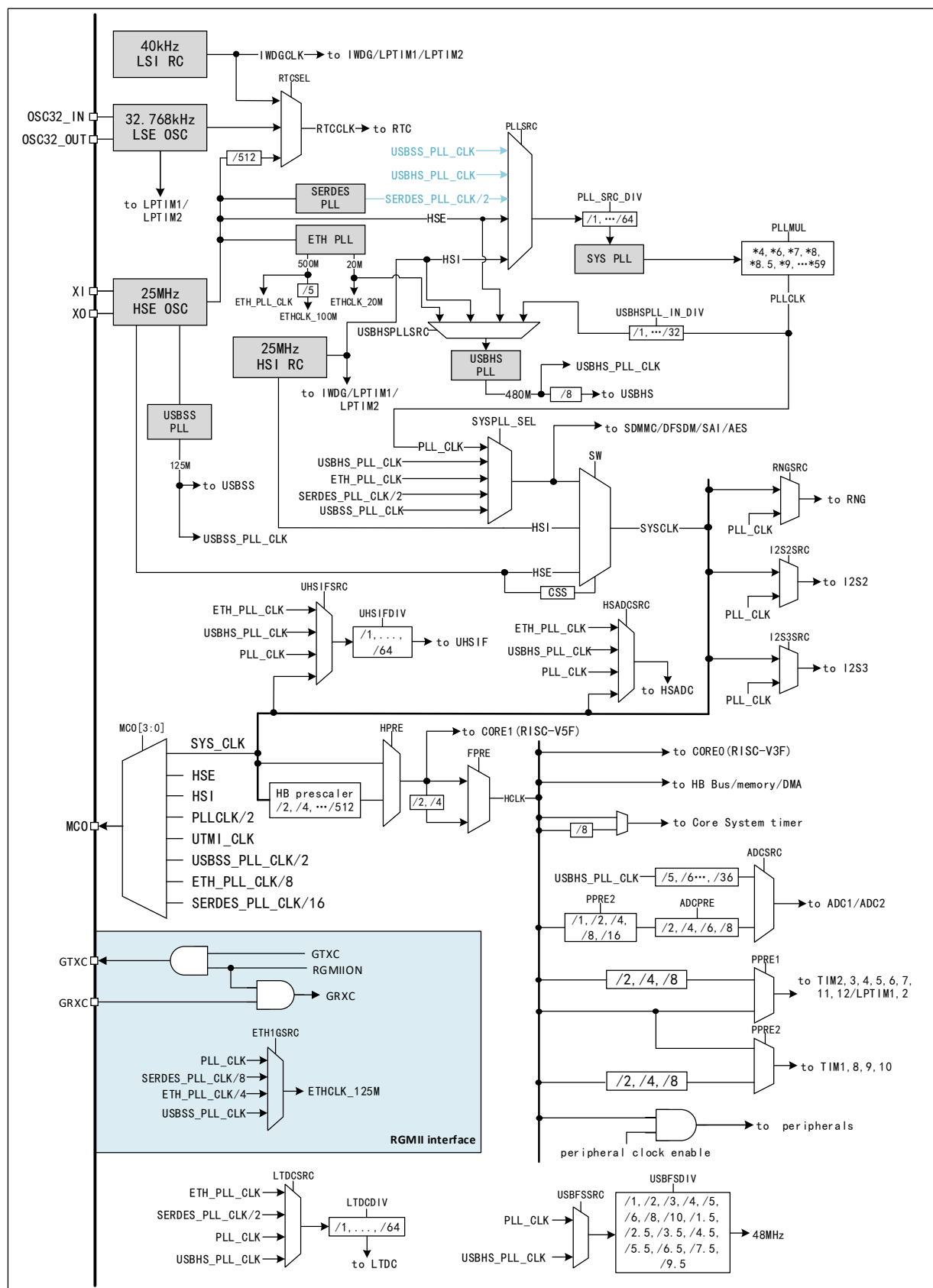
图 3-3 时钟树框图 (适用于批号第五位不为 0 的芯片)
