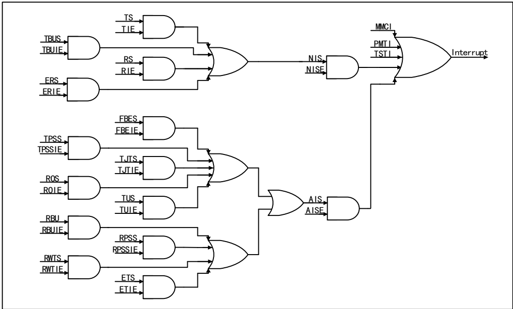
图 31-11 中断示意图
