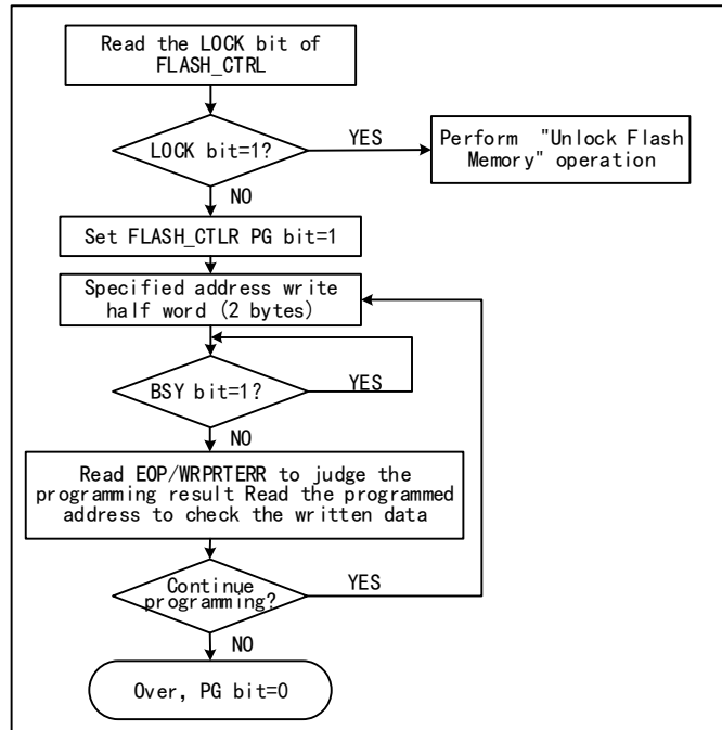
图 46-1 FLASH 编程
