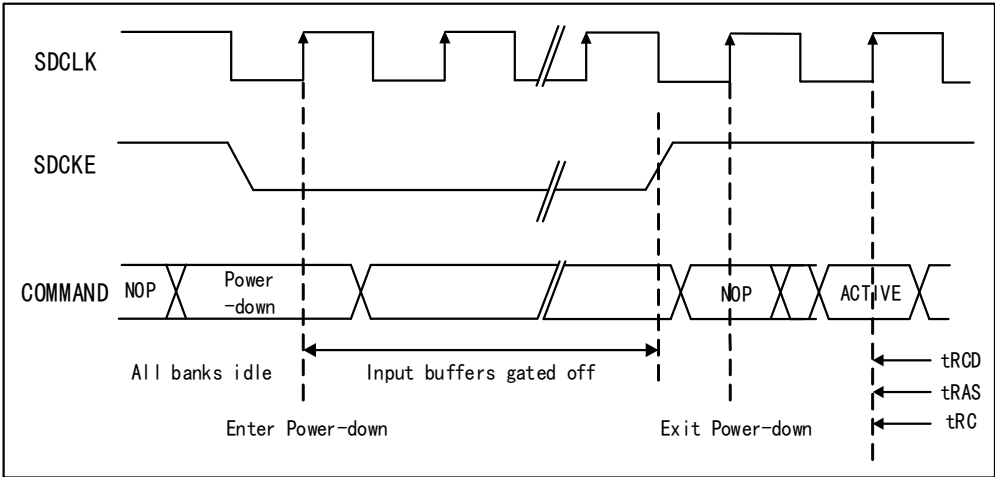
图 40-29 掉电模式
