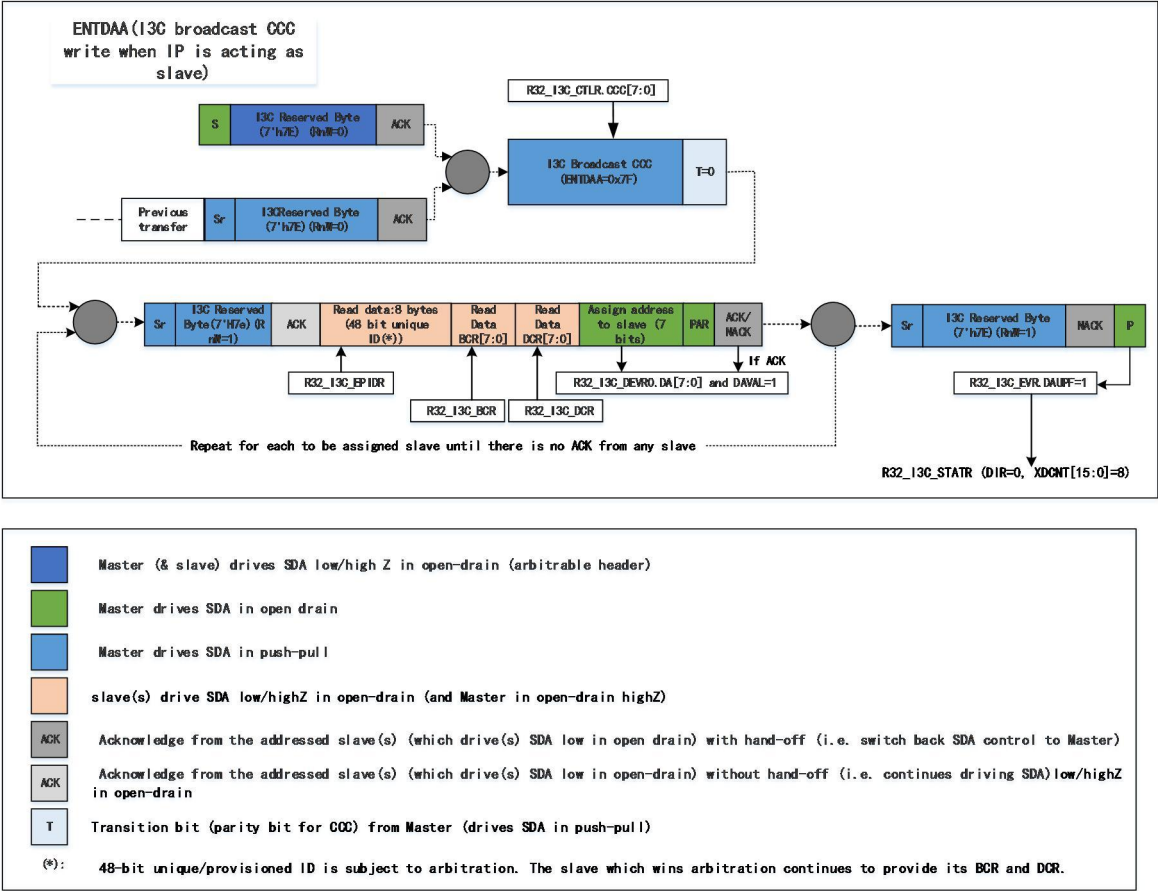
图 22-6 I3C 广播 ENTDAACCC 传输（作为从设备）
