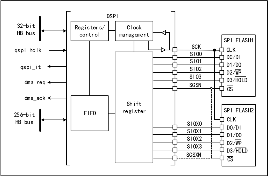
图 37-2 QSPI 功能框图（双闪存模式使能）
