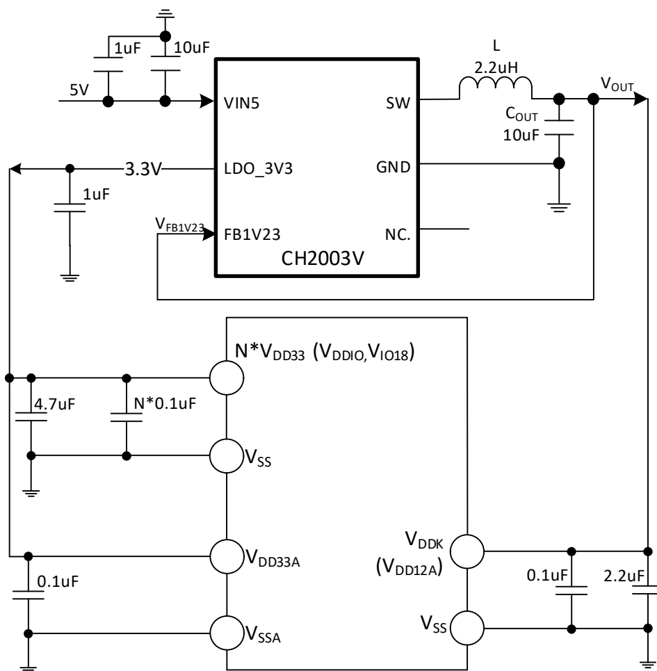
图 3-1-7 CH32H415 DCDC 单一 5V 供电电路
