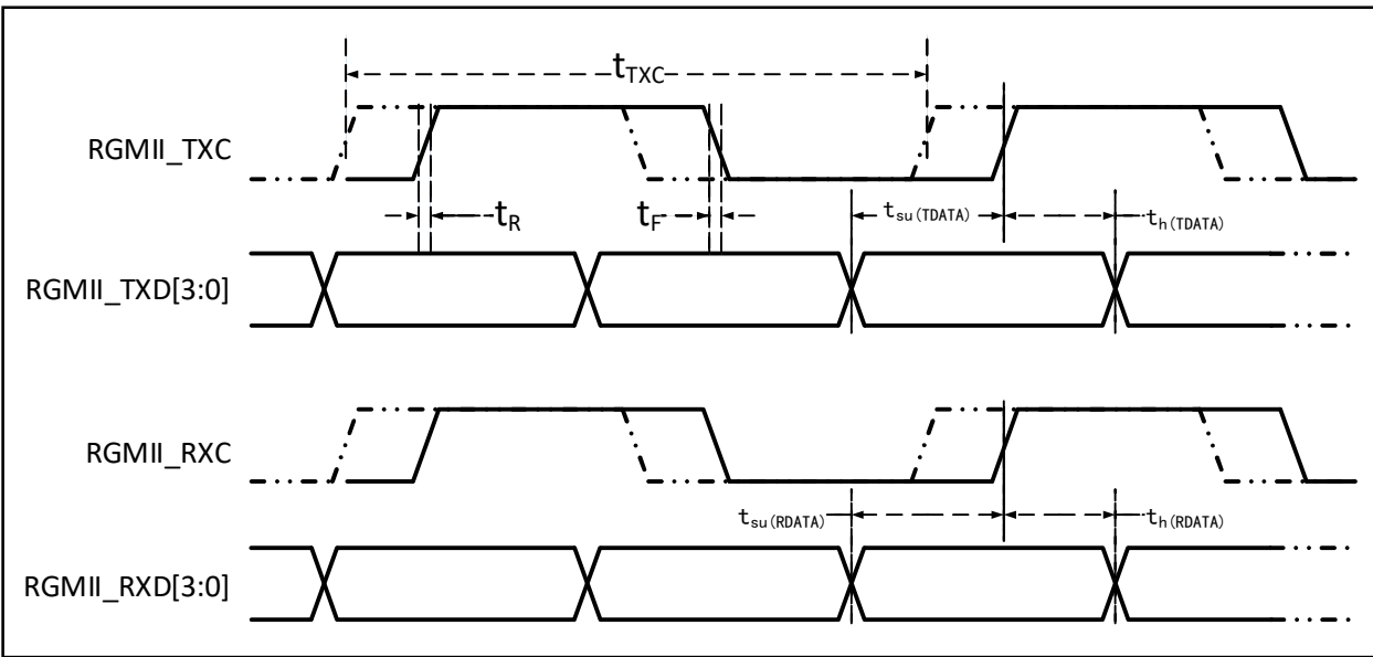
图 3-30 ETH-RGMII 信号时序波形
