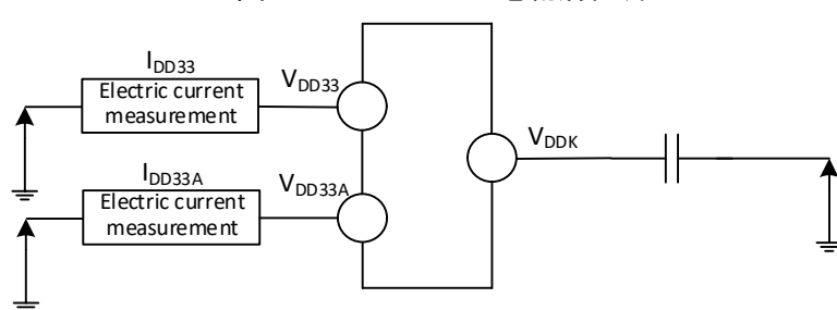
图 3-2-3 CH32H415 电流消耗测量
