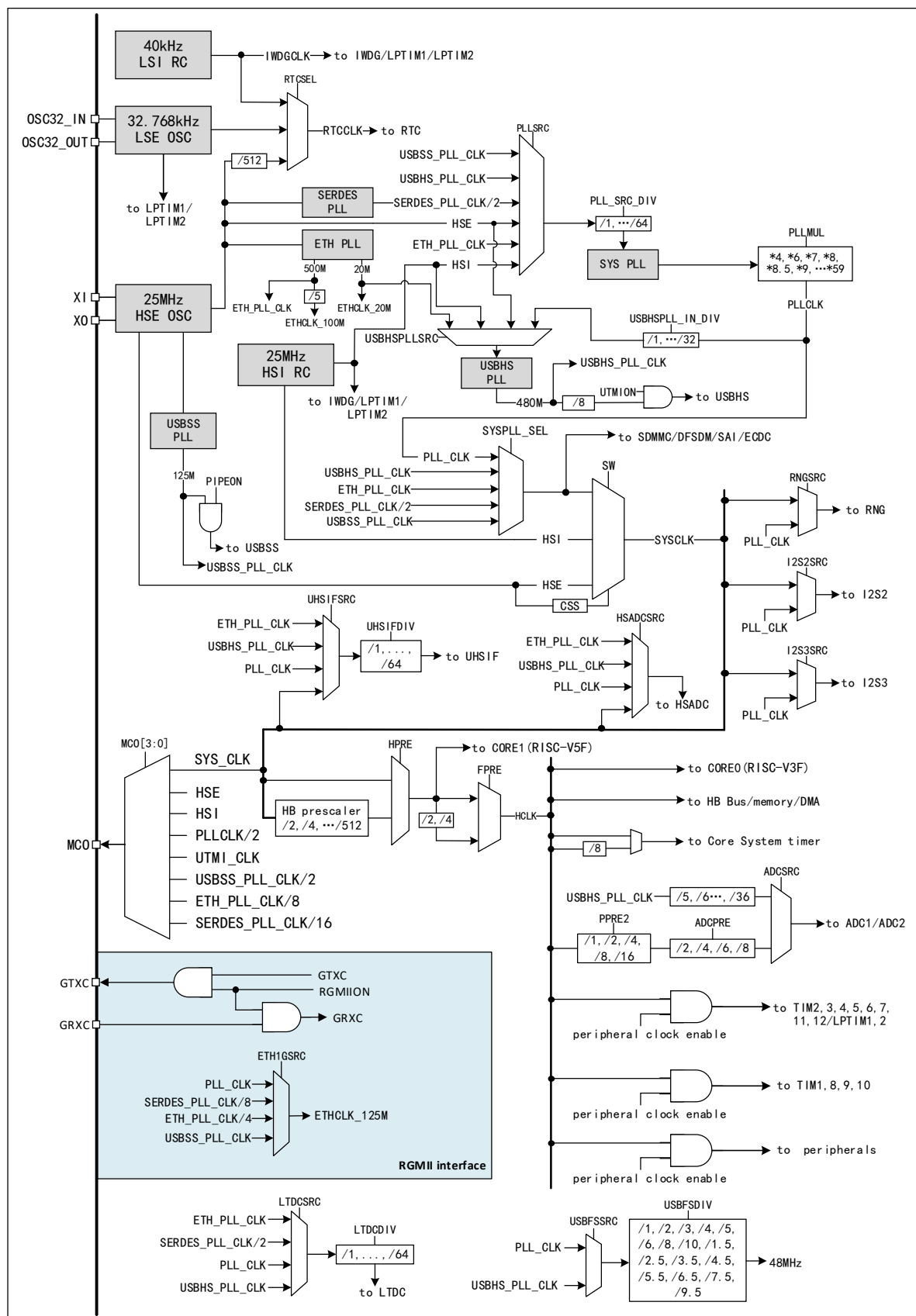
图 1-3 时钟树框图
