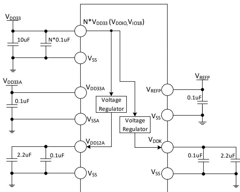
图 3-1-4 CH32H416 常规供电典型电路
