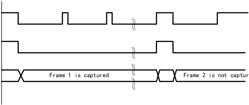
图 29-3 快照模式下的单帧捕获波形
