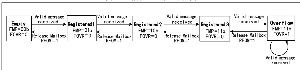
图 28-3 接收 FIFO 状态切换图
