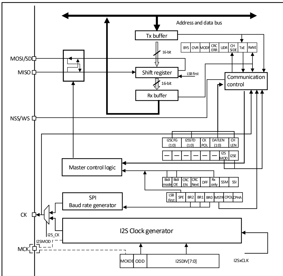
图 23-3 12S 结构框图
