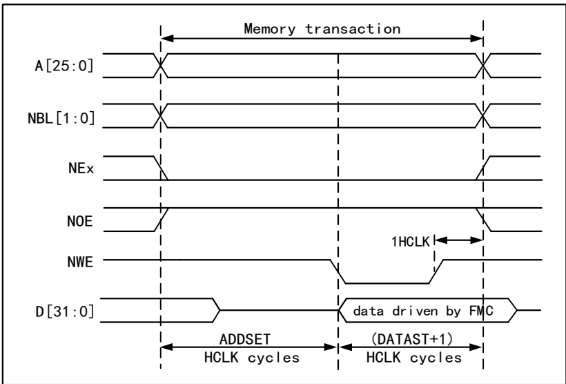
图 40-6 模式 A 写入访问波形
