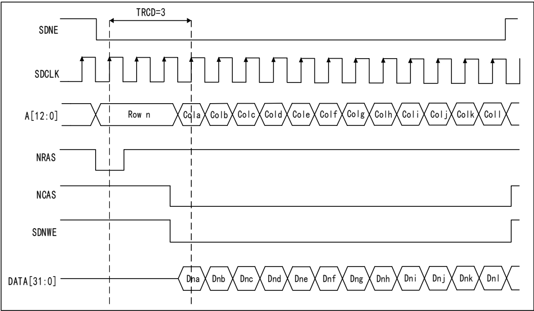
图 40-23 突发写入 SDRAM 访问波形
