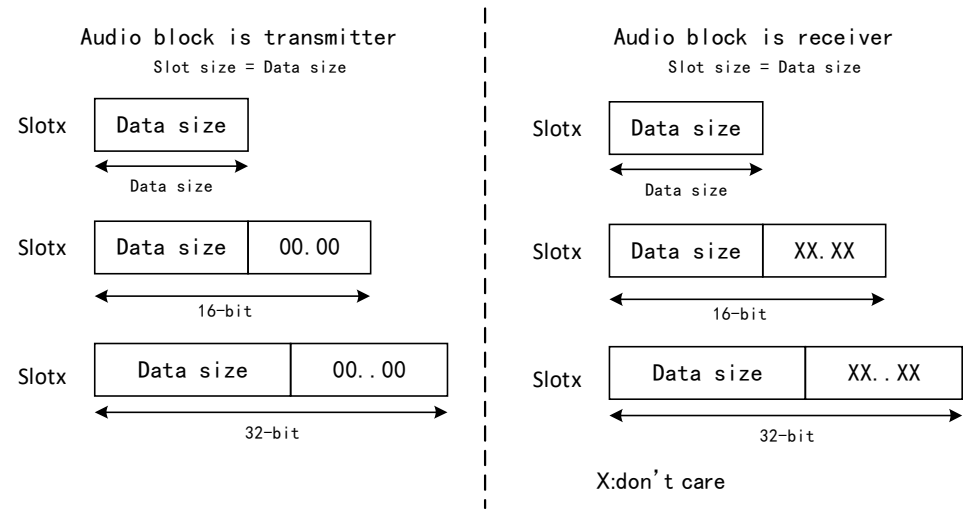
图 36-6 FBOFF 位为 0 时的 Slot 大小配置
