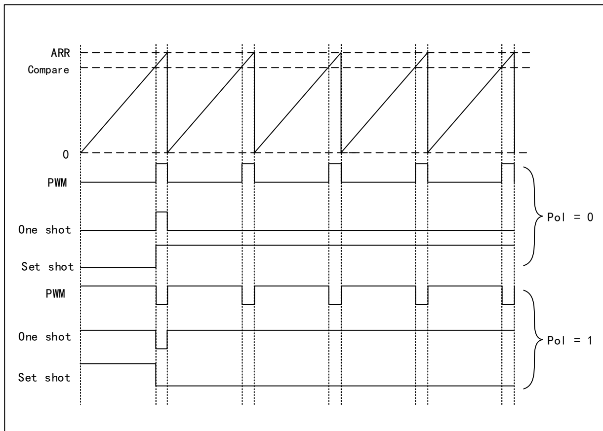
图 17-6 生成波形
