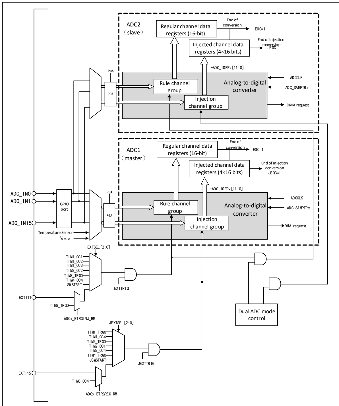
图 11-5 双 ADC 框图
