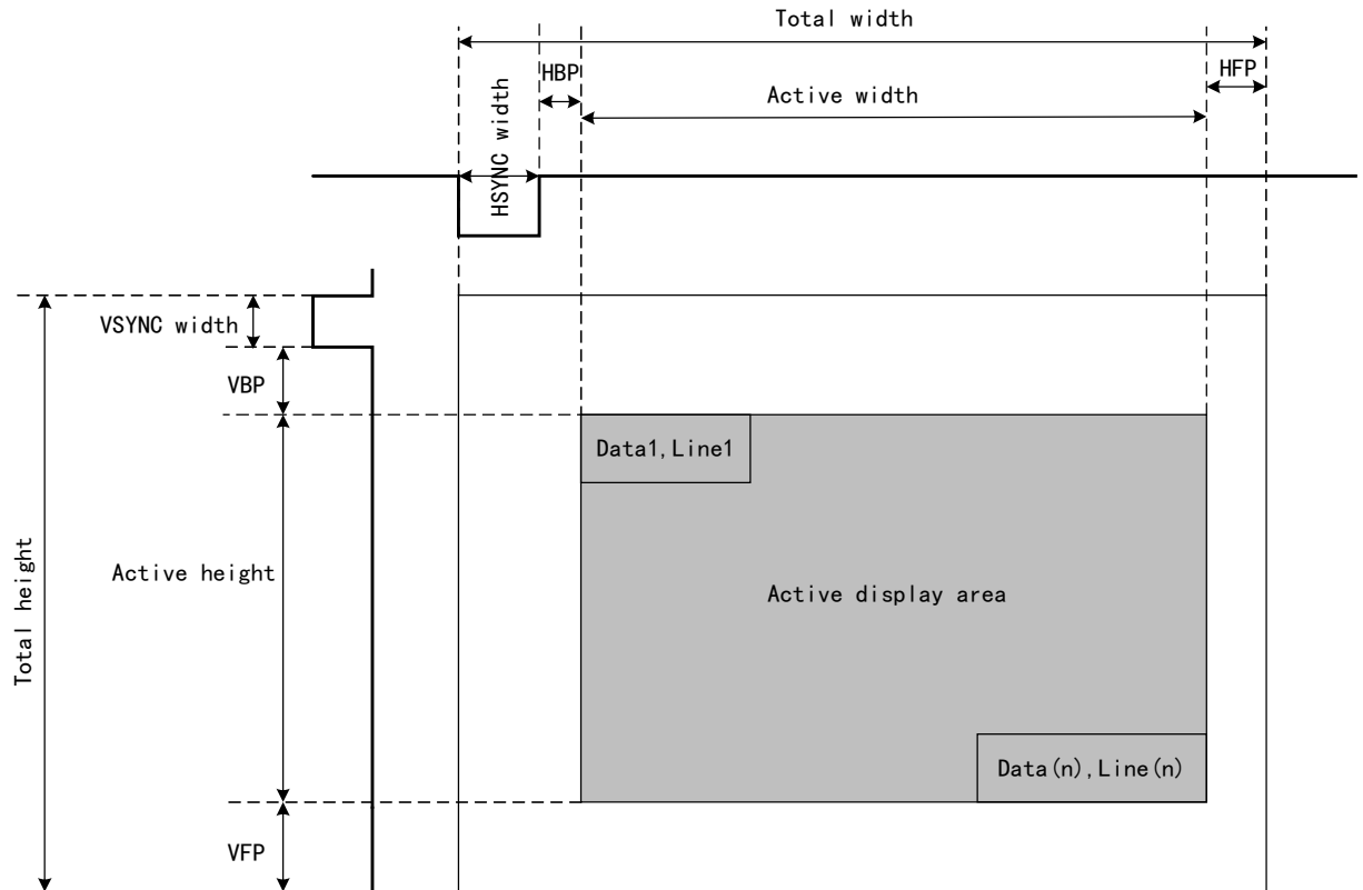
图 43-2 LTDC 同步时序
