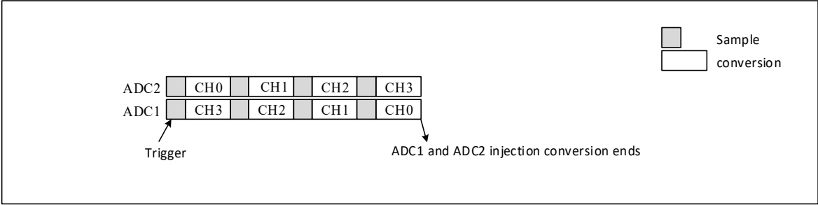
图 11-6 4 通道同步注入转换
