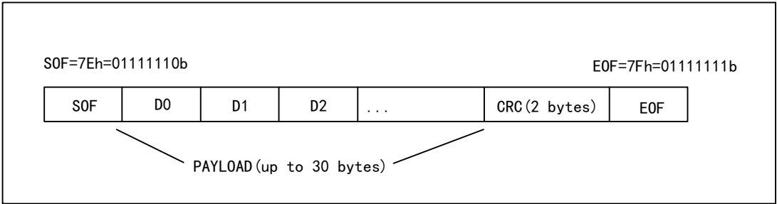
图 38-3 SWP 帧结构
