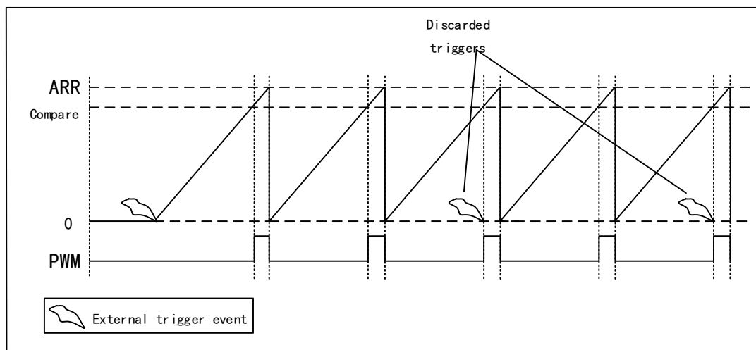
图 17-5 连续计数模式配置时的 LPTIM 输出波形
