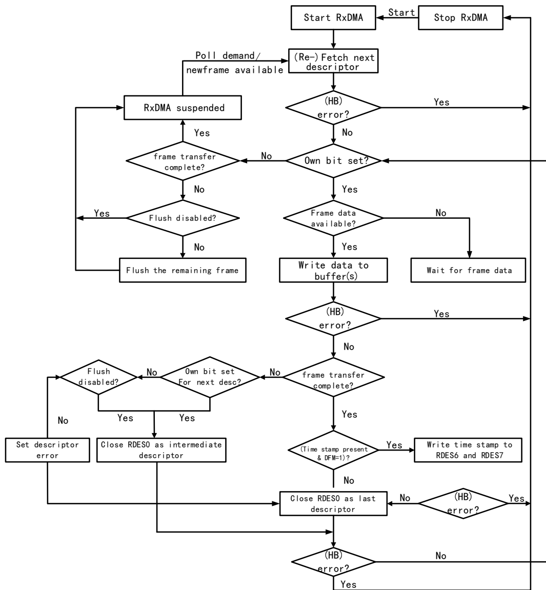
图 31-10 接收流程
