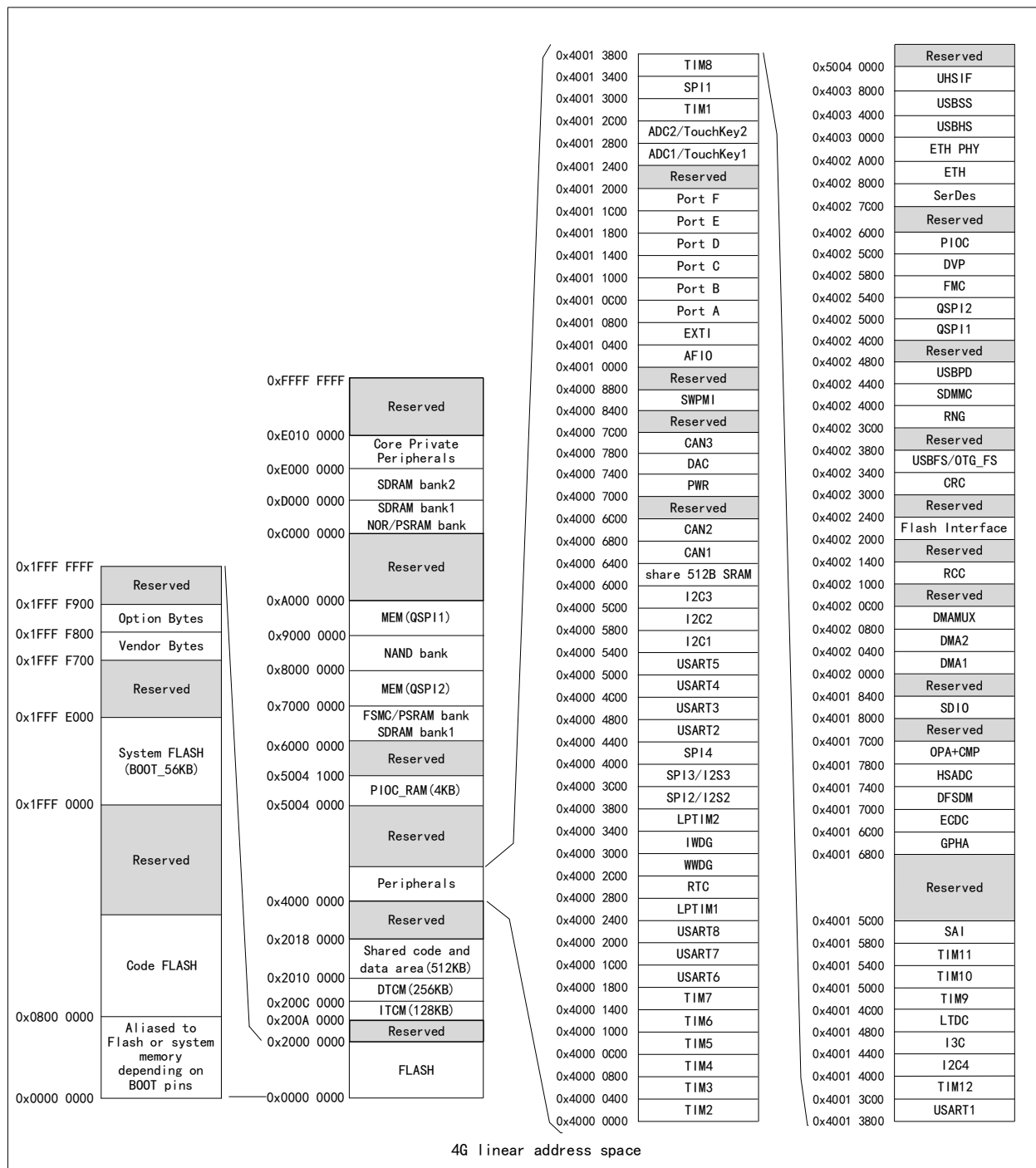
图 1-2 存储映像
