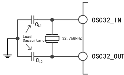
图 3-6 低速外部晶体电路
