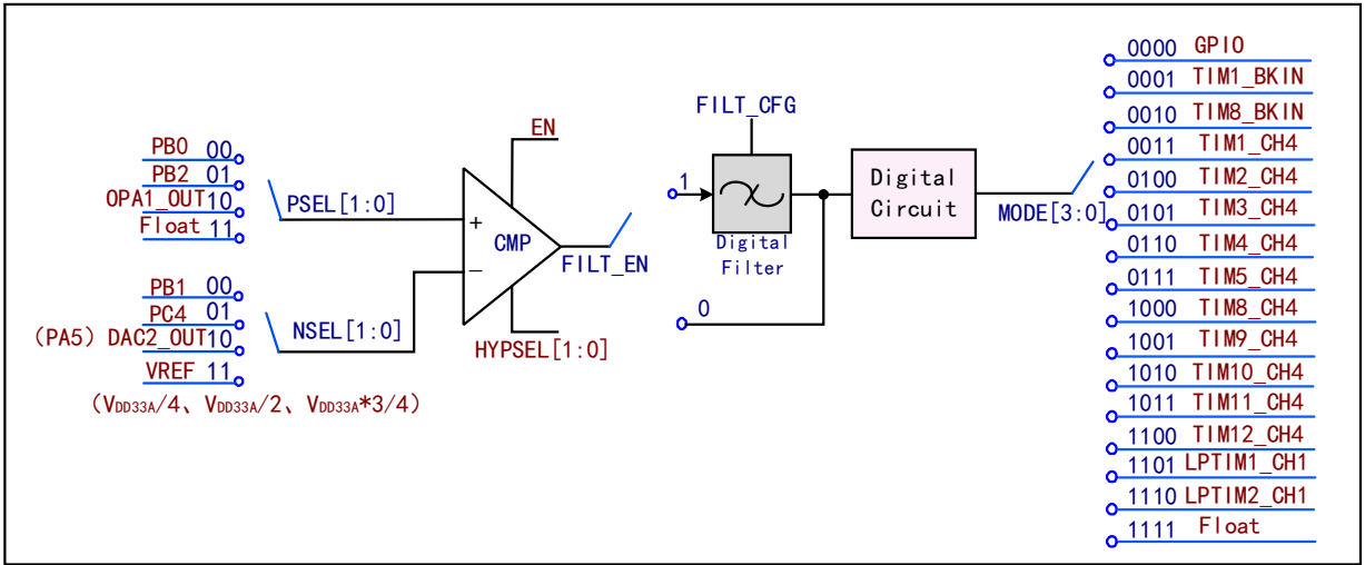
图 35-2 CMP 结构图
