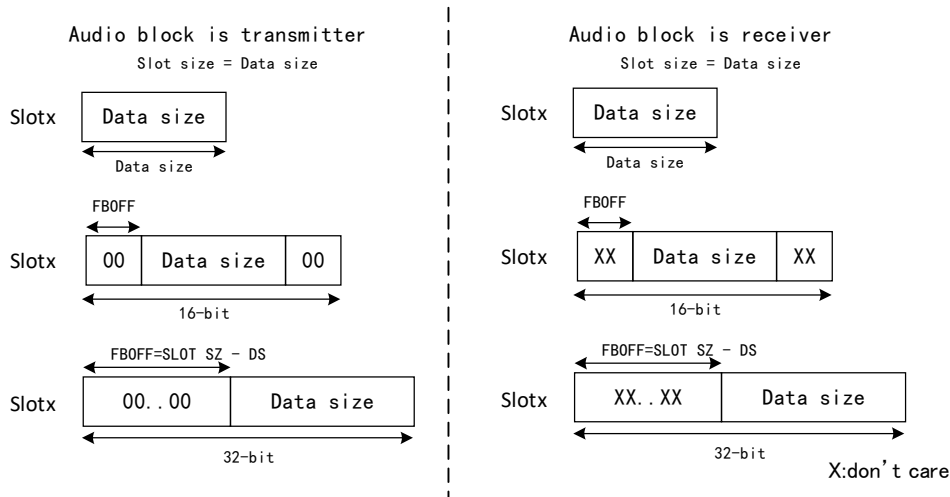
图 36-7 第一位偏移
