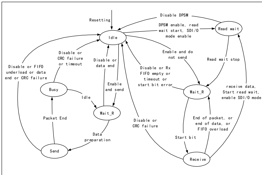
图 32-3 数据状态机
