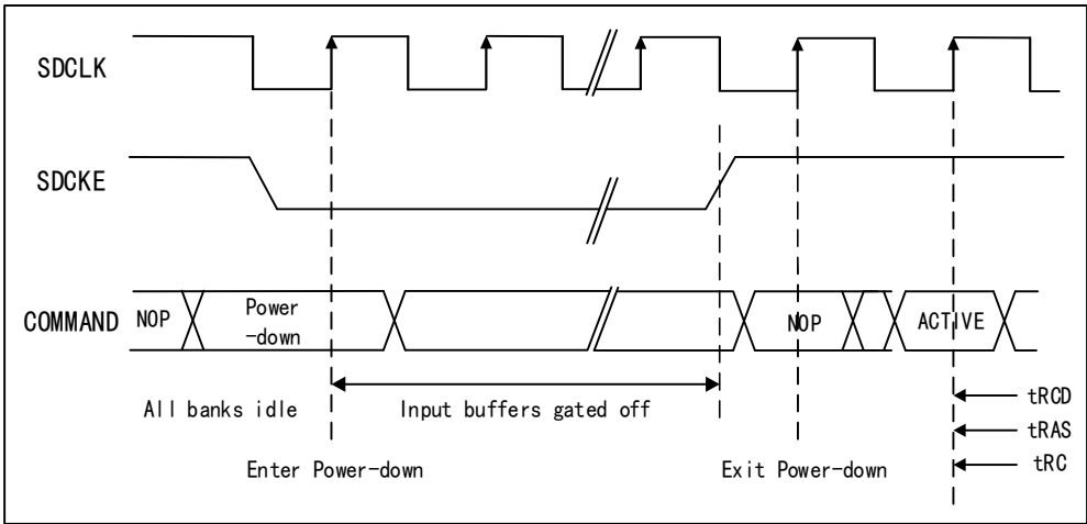
图 40-29 掉电模式
