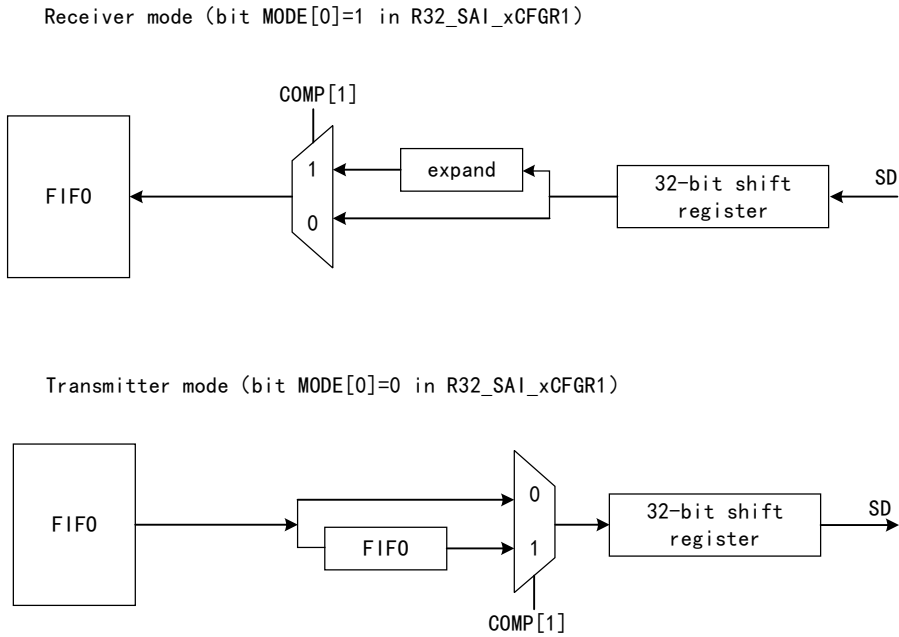
图 36-12 SAI 的音频模块中的数据压扩硬件
