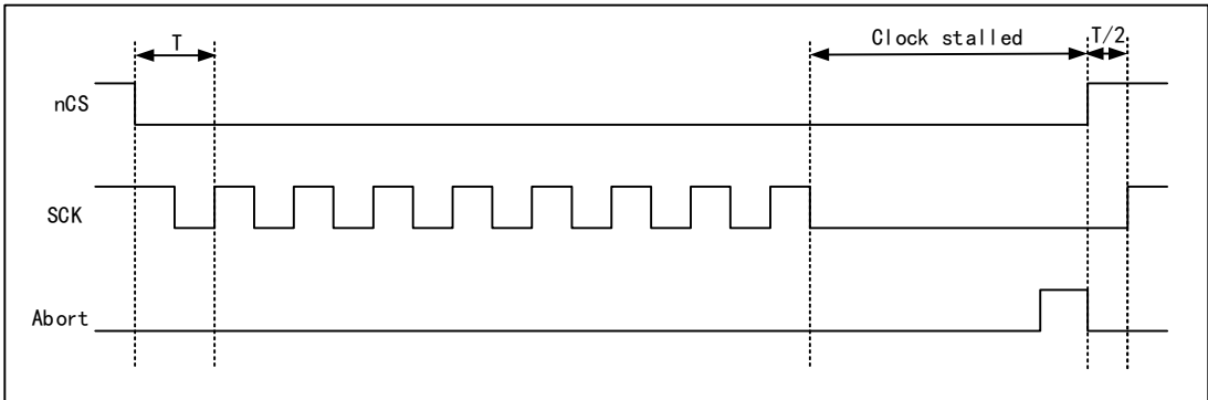
图 37-6 CKMODE=1 且发生中止时的 nCS（T=SCK 周期）
