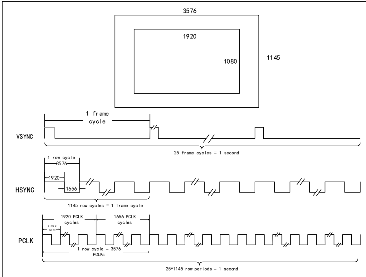
图 29-2 时序描述
