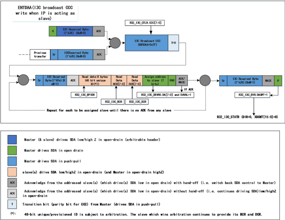
图 22-6 I3C 广播 ENTDAACCC 传输（作为从设备）
