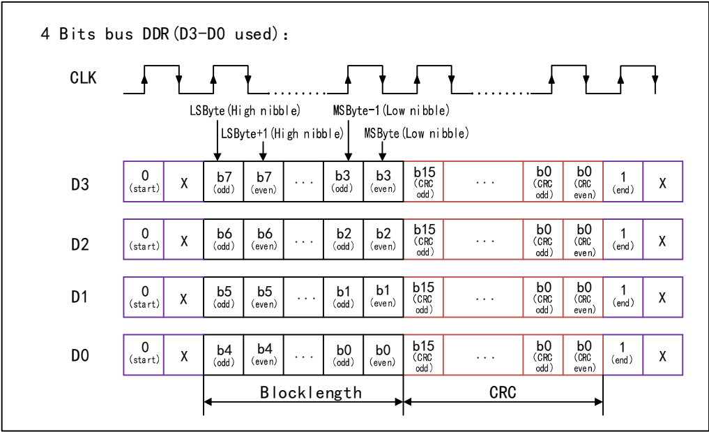
图 33-1 4 线的 DDR 模式
