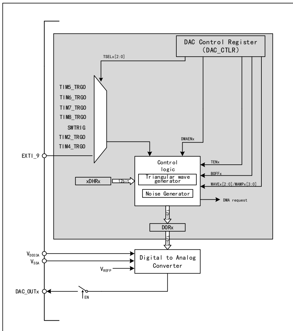
图 18-1 DAC 模块框图
