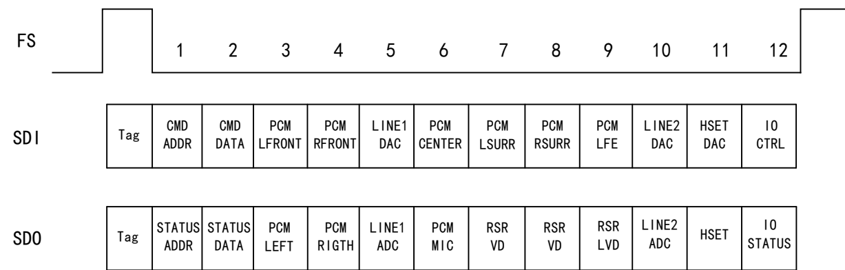
图 36-8 AC’ 97 音频帧
