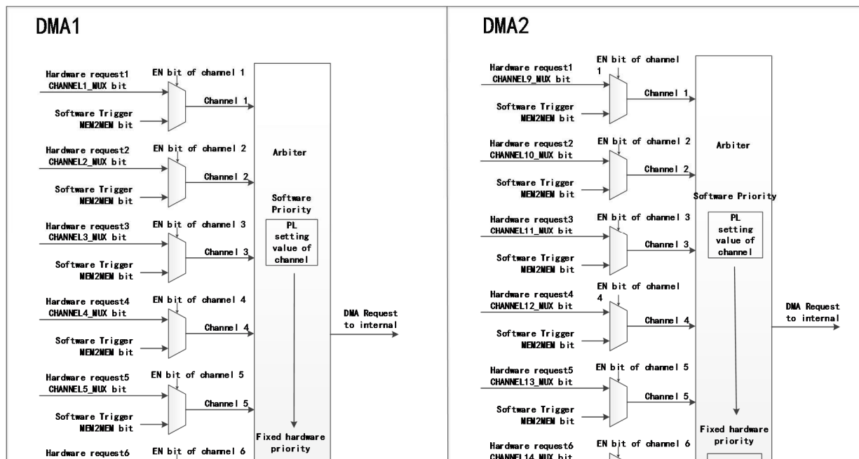
图 10-1 DMA 通道工作示意图
