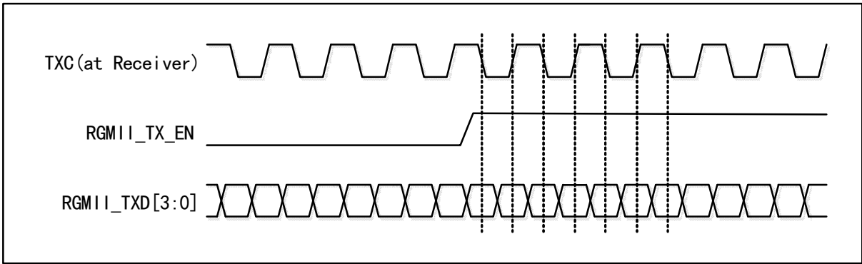
图 31-4 RGMII 的时序示意图
