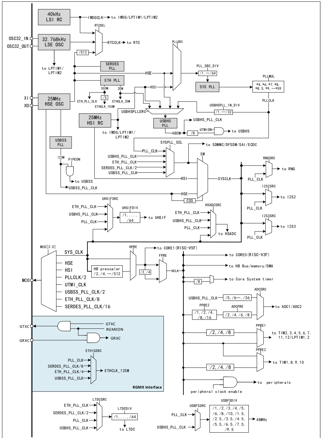
图 3-2 时钟树框图（仅适用于批号第五位为 0 的芯片）
