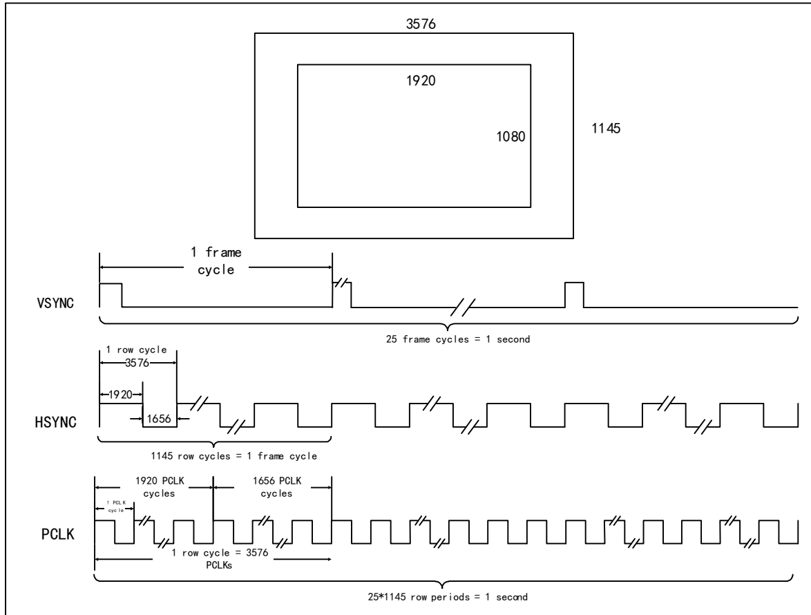
图 29-2 时序描述
