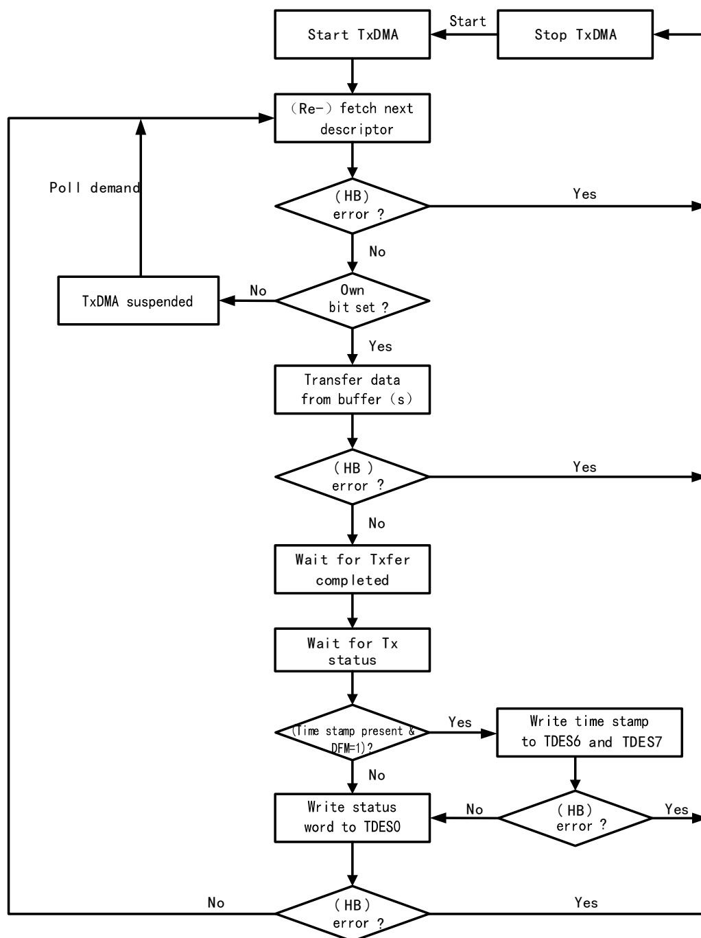
图 31-9 发送流程
