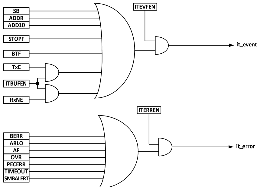
图 21-8 I2C 中断请求
