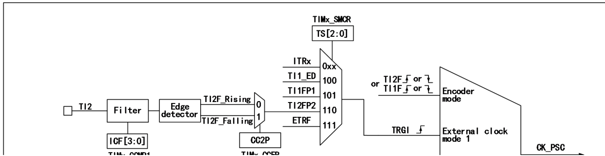
图 14-2 高级定时器的 CK_PSC 来源框图
