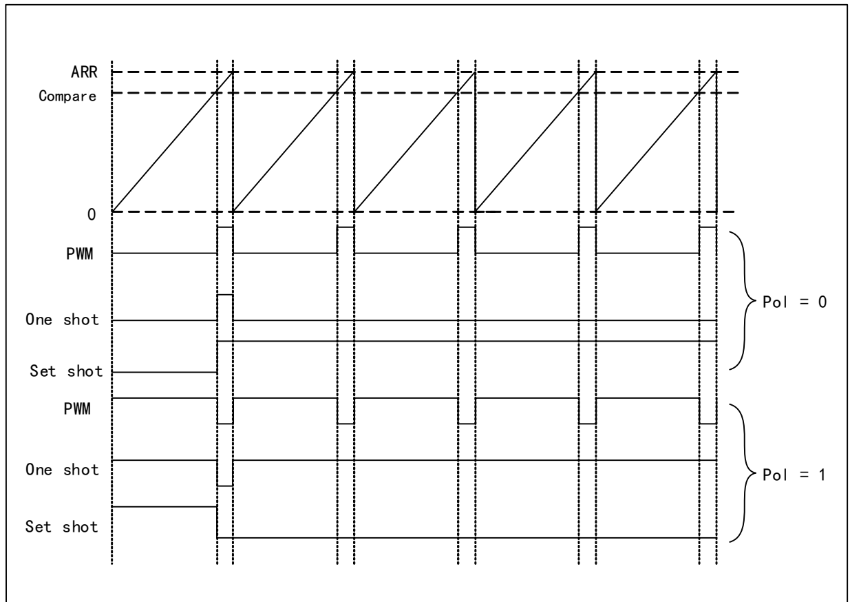
图 17-6 生成波形
