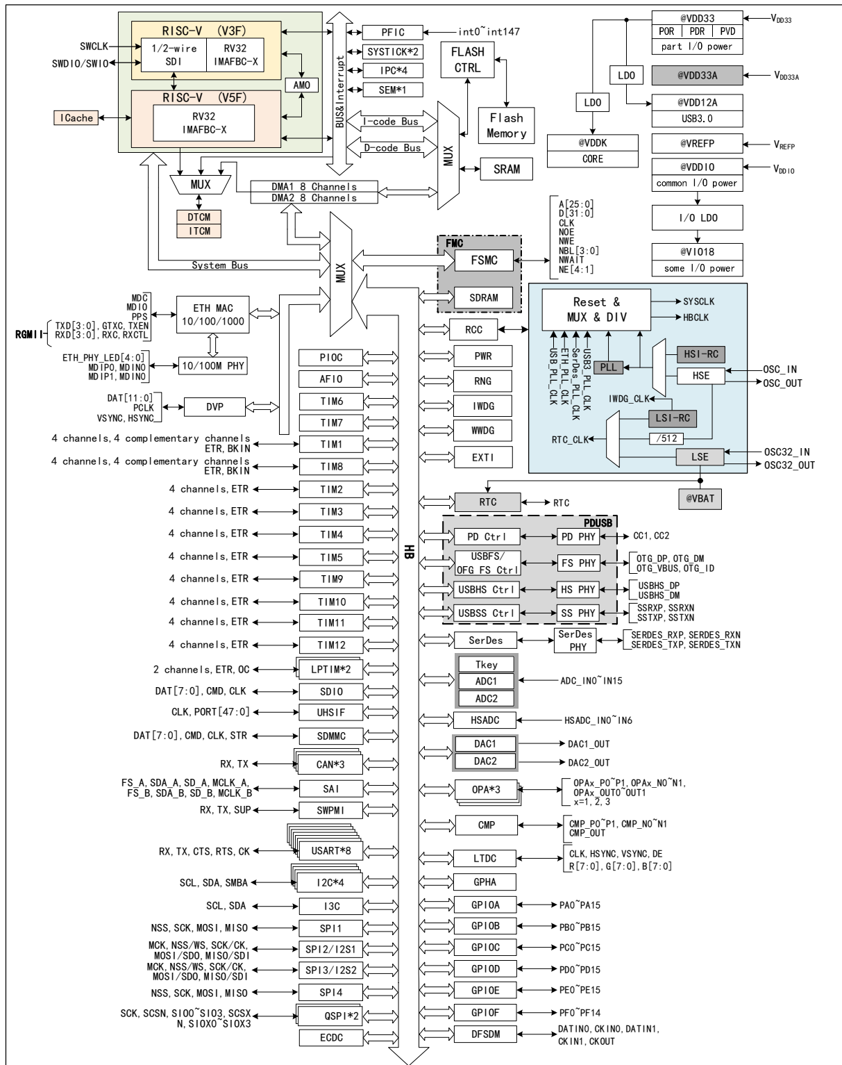
图 1-1 CH32H417 系统框图
