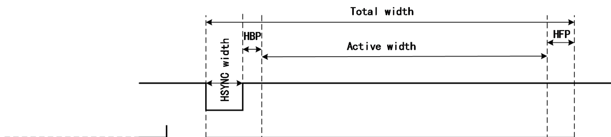
图 43-2 LTDC 同步时序
