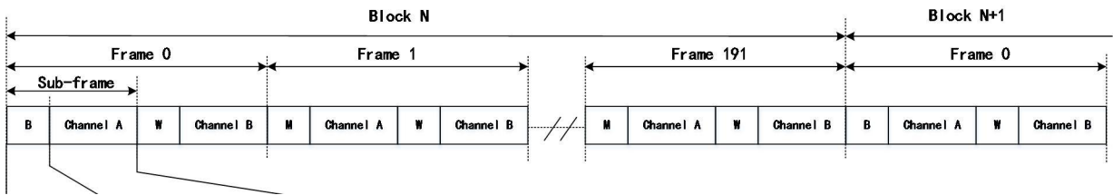
图 36-10 SPDIF 格式
