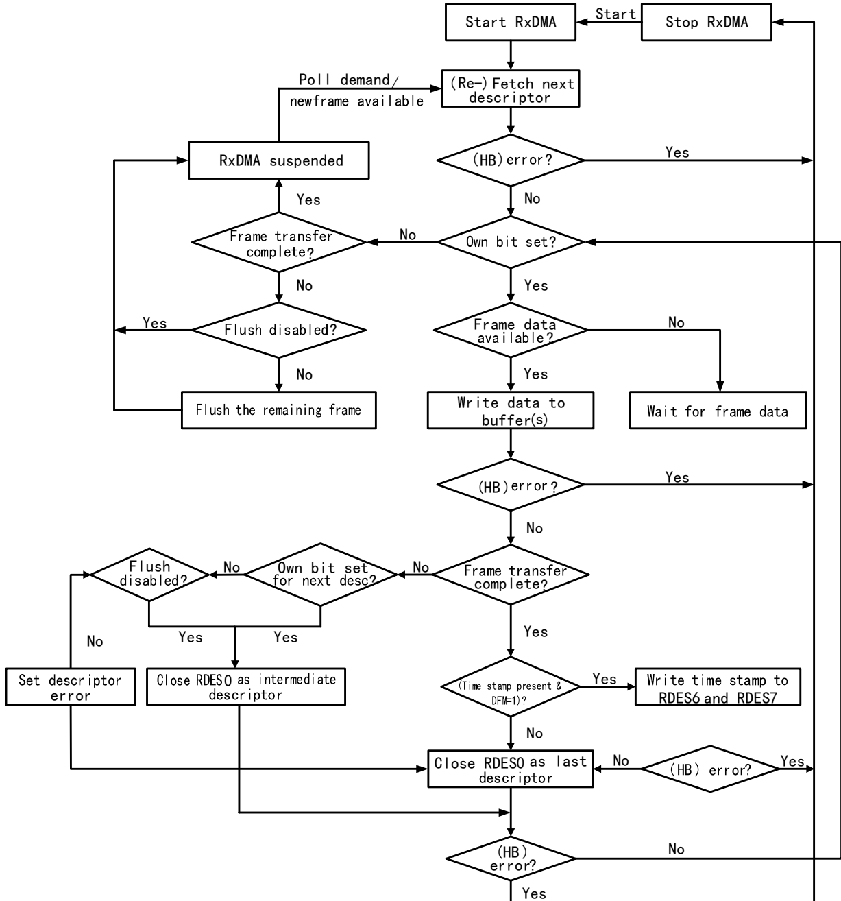
图 31-10 接收流程
