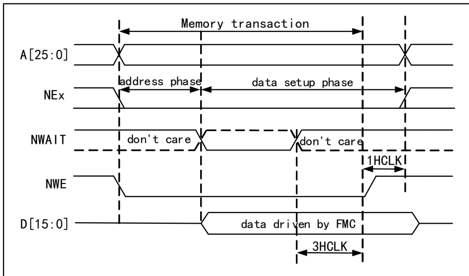
图 40-17 写入访问波形期间的异步等待
