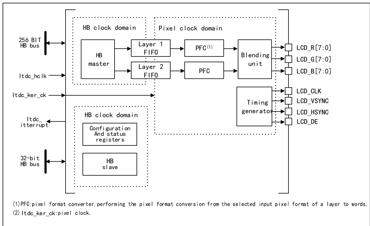
图 43-1 LTDC 结构框图
