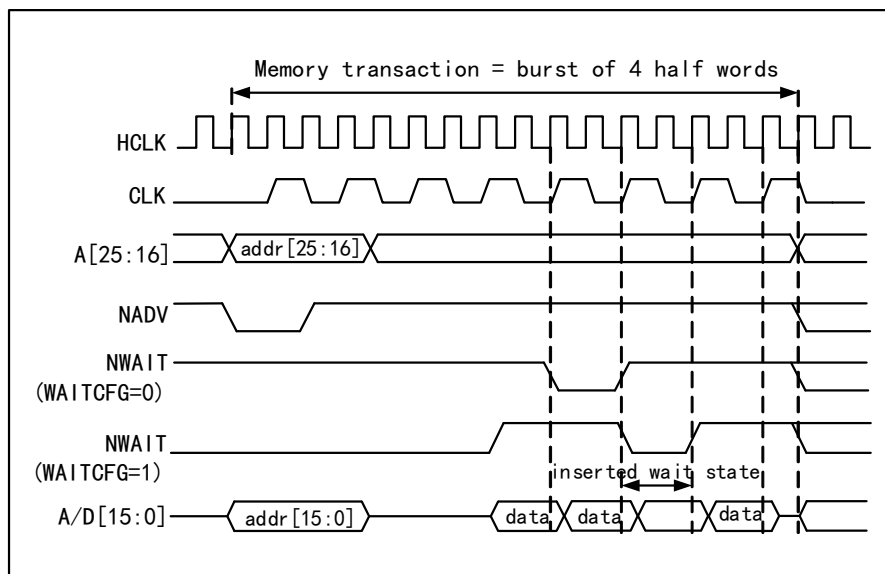
图 40-18 等待配置波形
