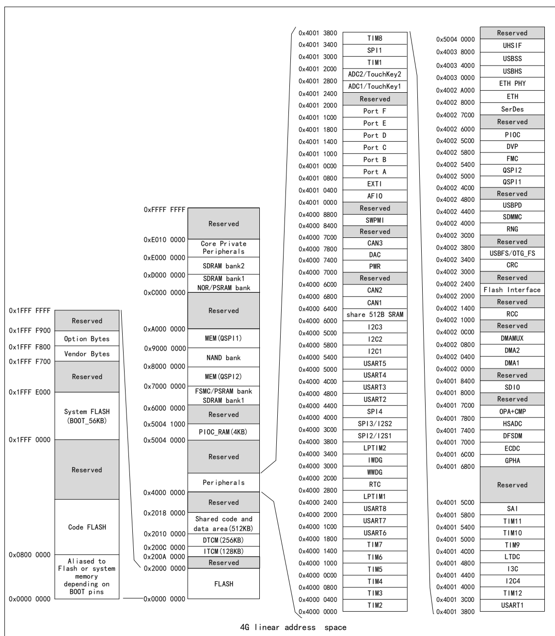
图 1-2 CH32H417 存储映像
