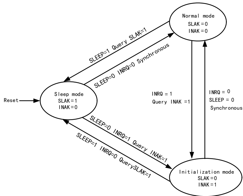
图 28-1 CAN 工作模式切换
