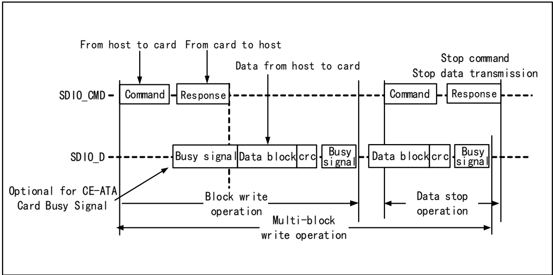
图 32-6 SDIO 的多块写时序（以 SD 卡为例）
