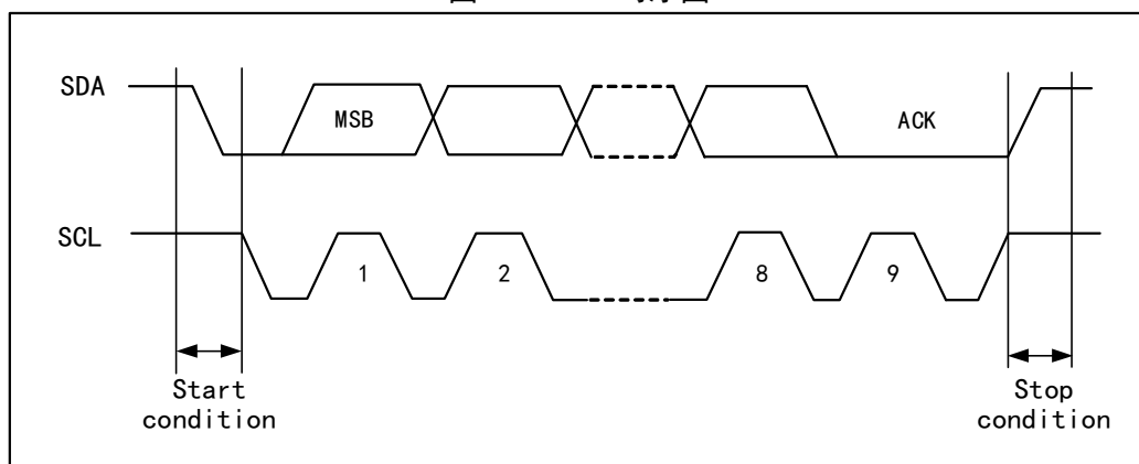
图 21-1 I2C 时序图
