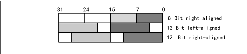
图 18-3 双通道数据格式
