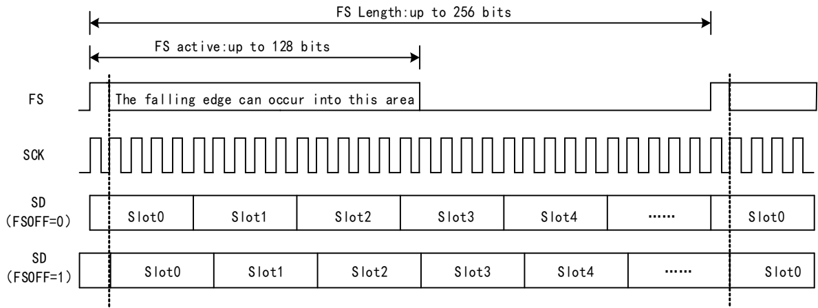
图 36-3 音频帧
