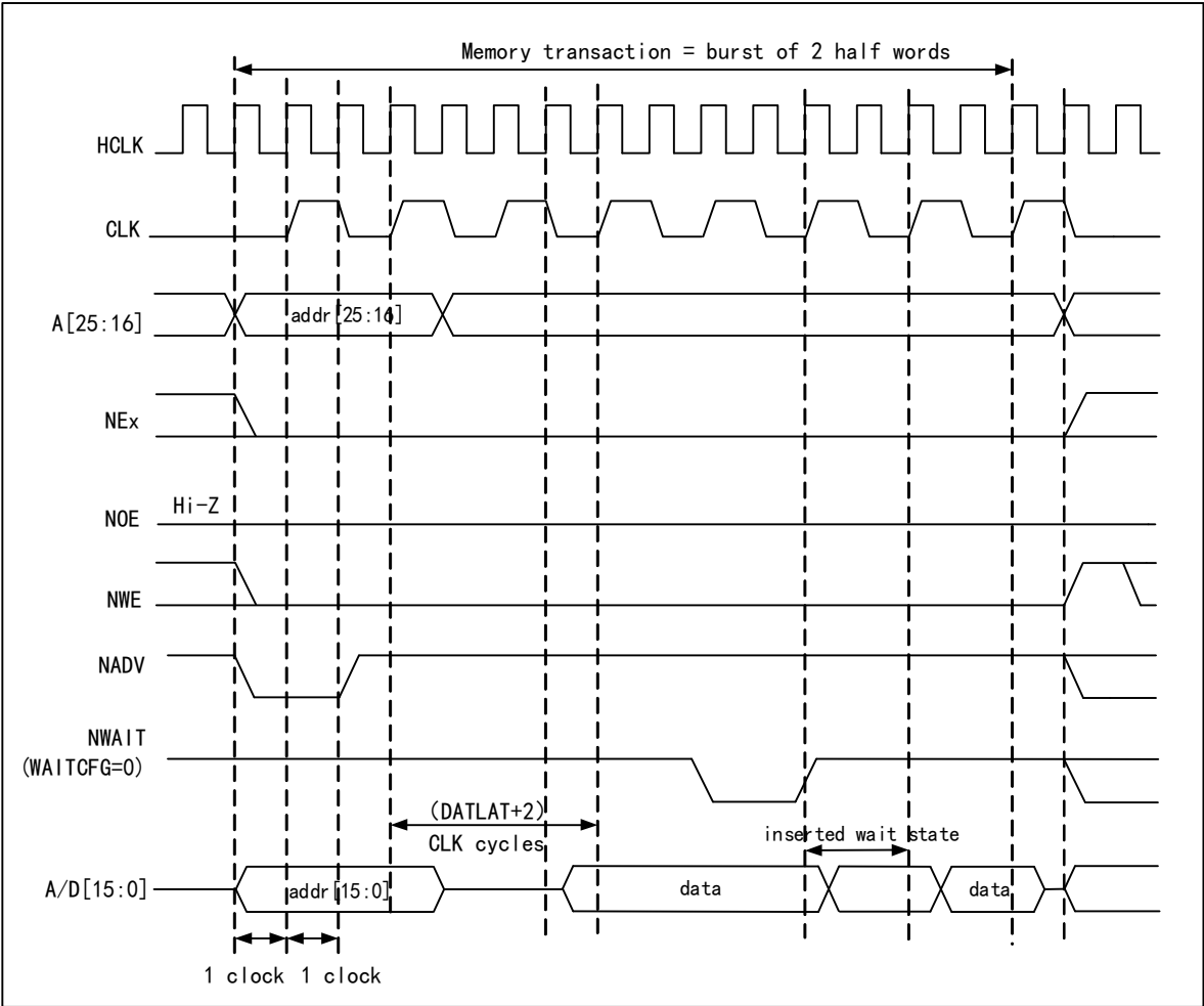
图 40-20 同步复用写入模式波形-PSRAM（GRAM）
