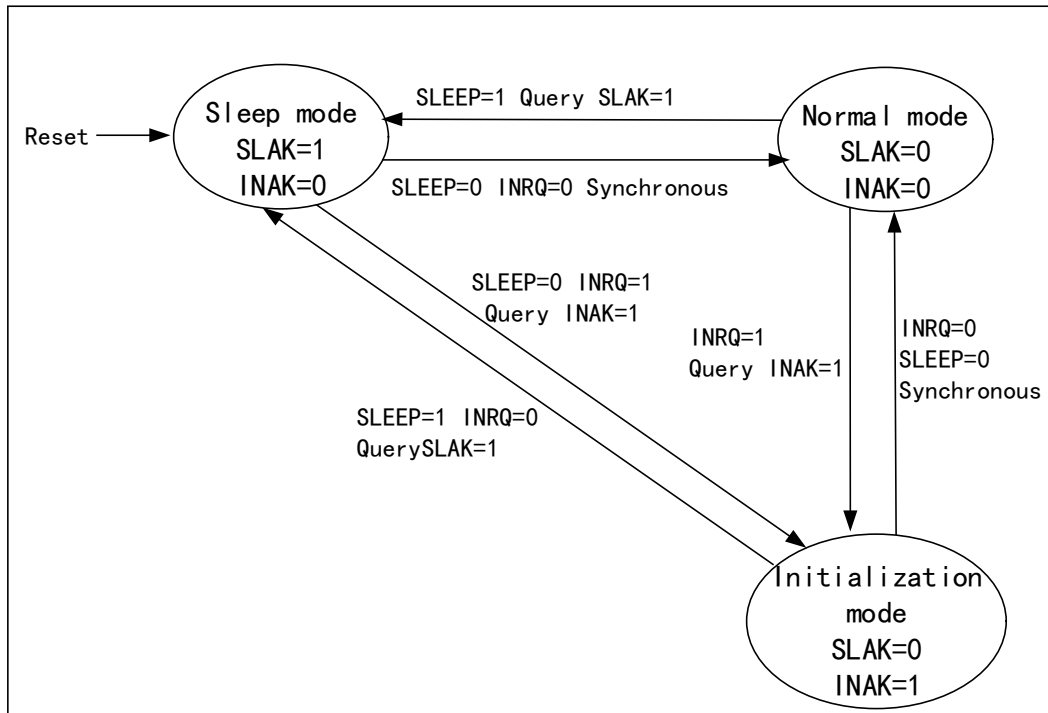
图 22-1 CAN 工作模式切换
