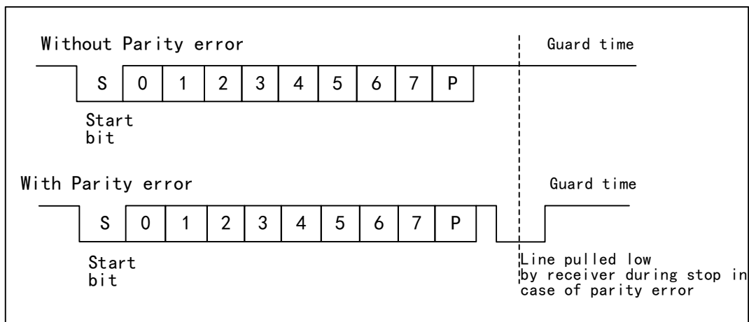
图 17-4（未）发生奇偶校验错误示意图
