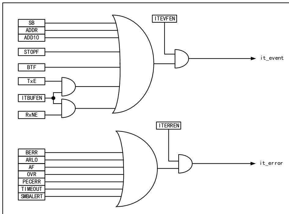
图 18-4 I2C 中断请求
