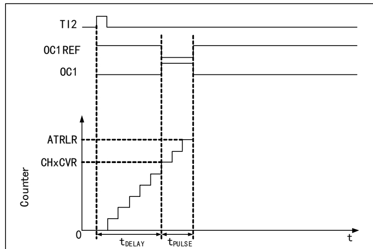
图 15-4 事件产生和脉冲响应
