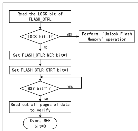
图 24-2 FLASH 整片擦除
